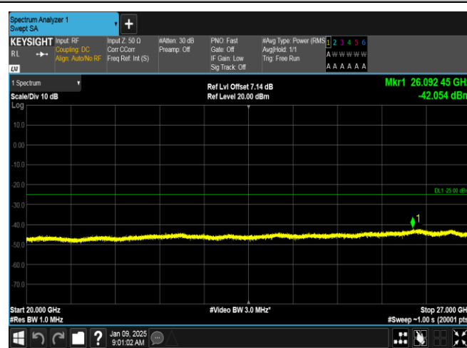
Band38-5MHz-QPSK-38000-25RB#0-20000~27000-PASS
