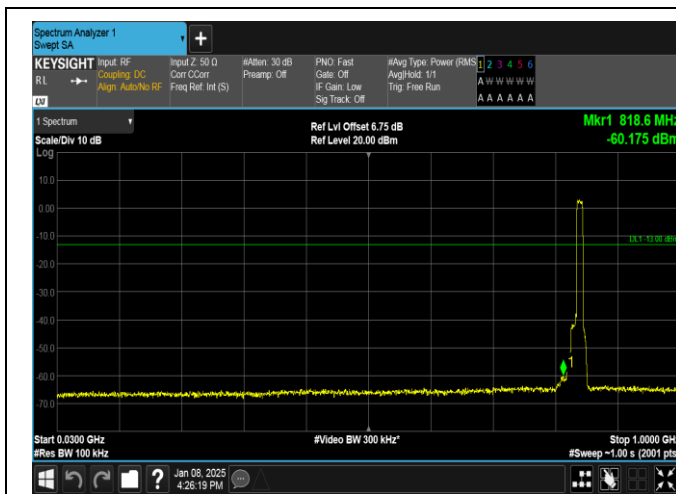
Band26(824-849)-10MHz-QPSK-26990-50RB#0-30~1000-PASS
