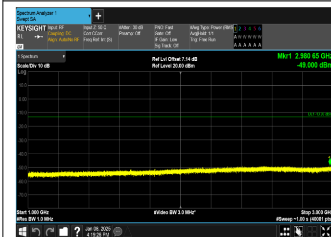
Band26(824-849)-10MHz-QPSK-26915-50RB#0-1000~3000-PASS
