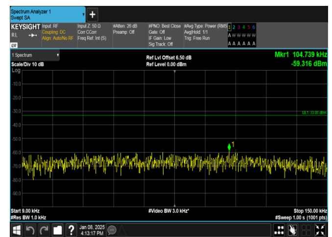
Band26(824-849)-10MHz-QPSK-26915-1RB#0-0.009~0.15-PASS
