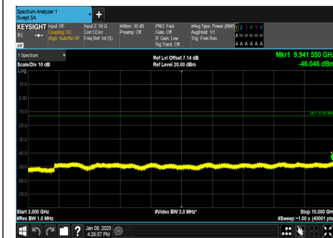
Band26(824-849)-10MHz-QPSK-26990-50RB#0-3000~10000-PASS
