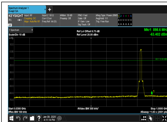
Band26(824-849)-10MHz-QPSK-26840-50RB#0-30~1000-PASS
