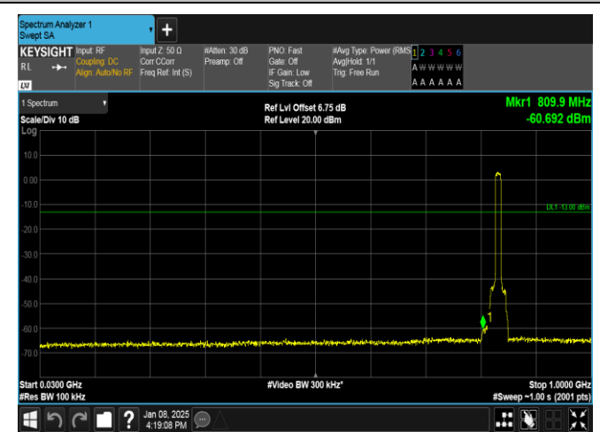
Band26(824-849)-10MHz-QPSK-26915-50RB#0-30~1000-PASS
