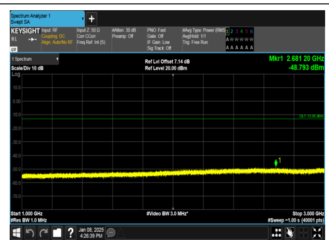
Band26(824-849)-10MHz-QPSK-26990-50RB#0-1000~3000-PASS
