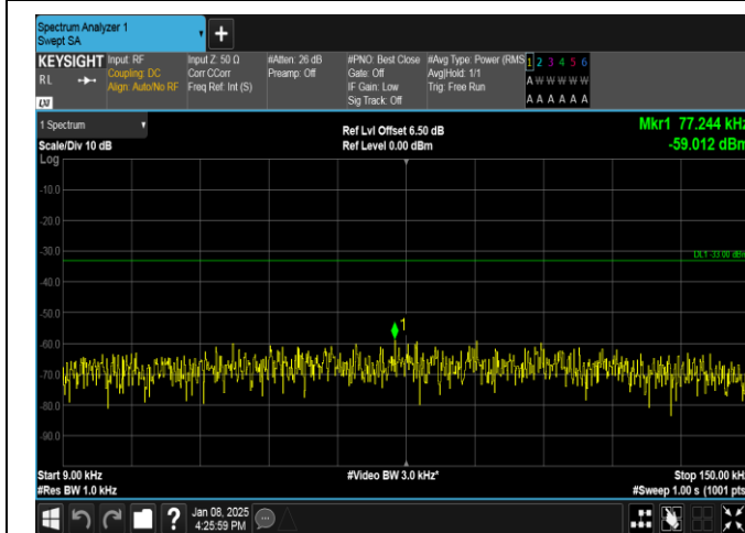
Band26(824-849)-10MHz-QPSK-26990-50RB#0-0.009~0.15-PASS
