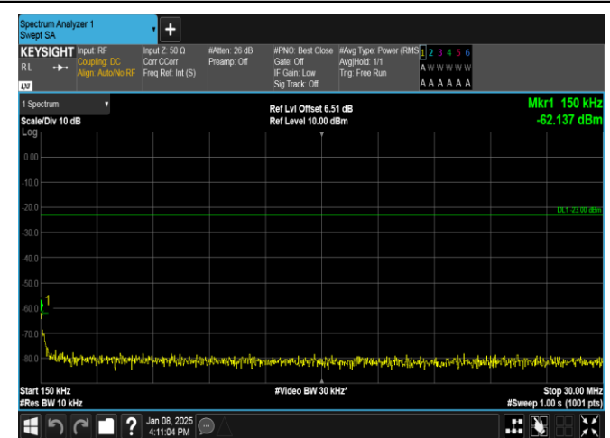
Band26(824-849)-10MHz-QPSK-26840-50RB#0-0.15~30-PASS
