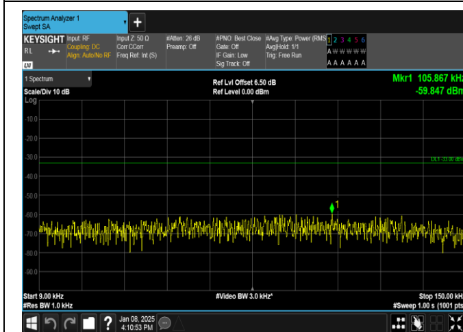
Band26(824-849)-10MHz-QPSK-26840-50RB#0-0.009~0.15-PASS
