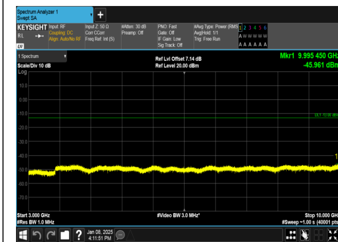
Band26(824-849)-10MHz-QPSK-26840-50RB#0-3000~10000-PASS
