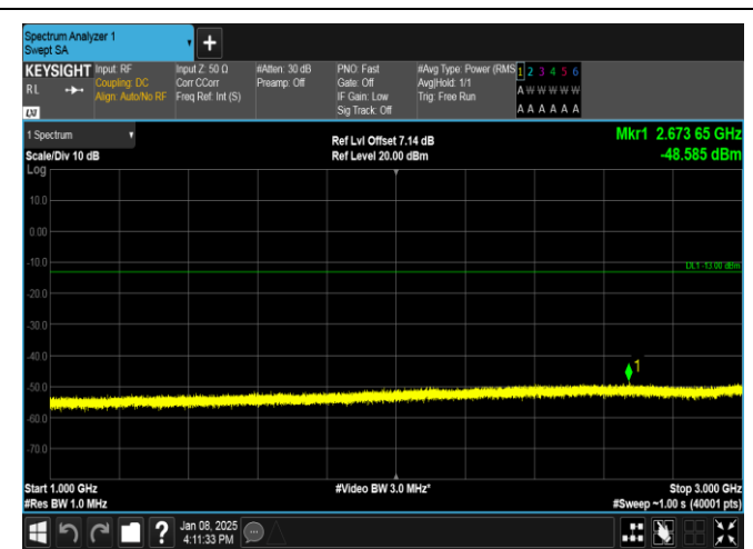
Band26(824-849)-10MHz-QPSK-26840-50RB#0-1000~3000-PASS
