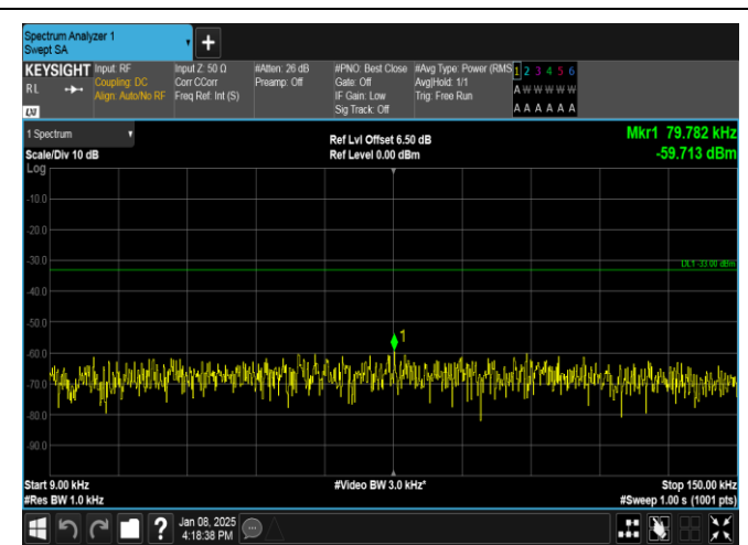
Band26(824-849)-10MHz-QPSK-26915-50RB#0-0.009~0.15-PASS
