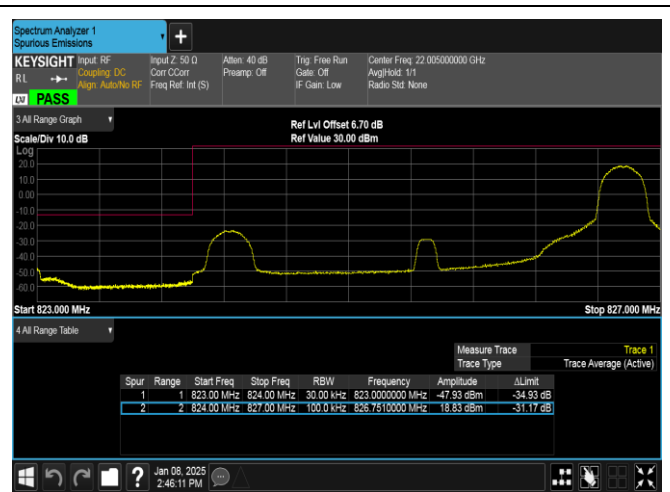
Band26(824-849)-3MHz-QPSK-26805-1RB#14-PASS
