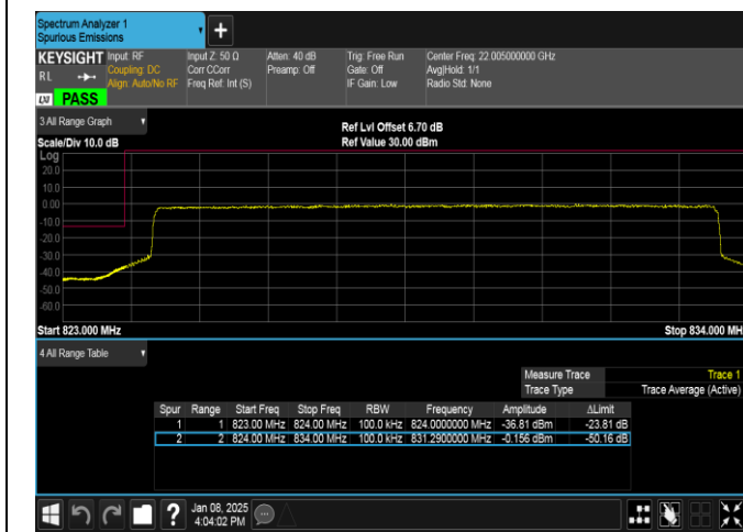
Band26(824-849)-10MHz-QPSK-26840-50RB#0-PASS
