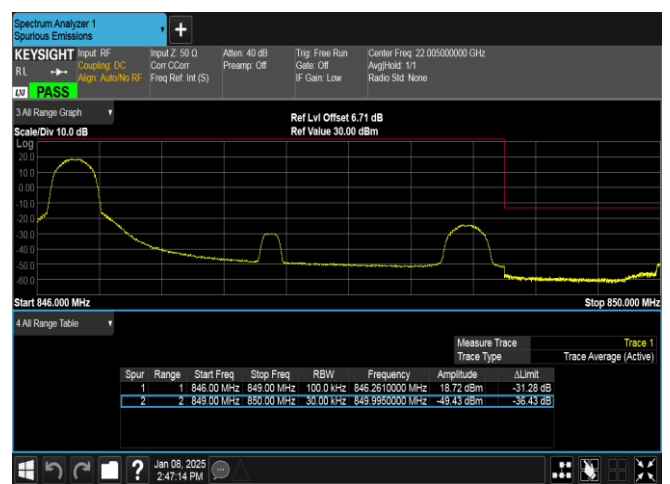
Band26(824-849)-3MHz-QPSK-27025-1RB#0-PASS
