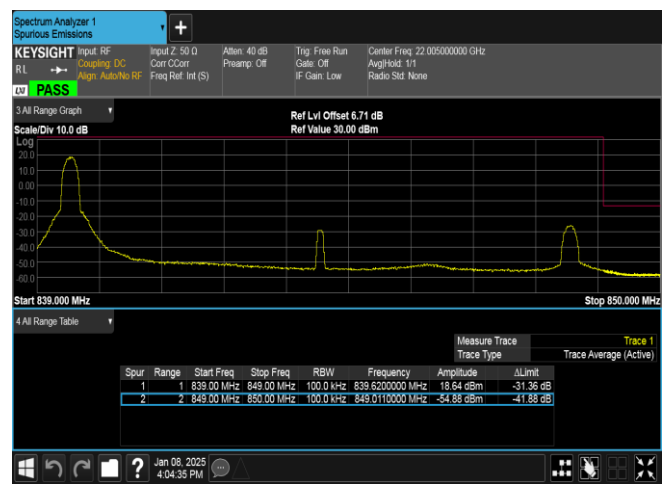
Band26(824-849)-10MHz-QPSK-26990-1RB#0-PASS
