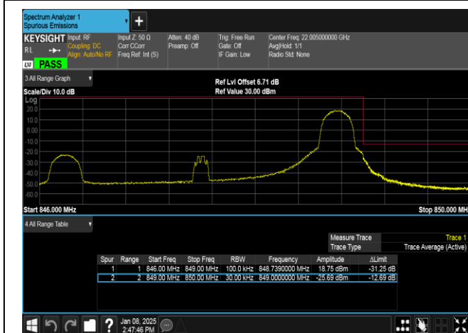
Band26(824-849)-3MHz-QPSK-27025-1RB#14-PASS
