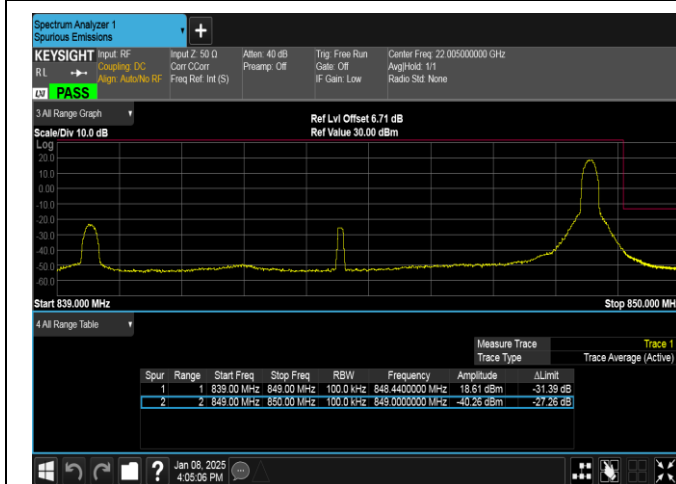
Band26(824-849)-10MHz-QPSK-26990-1RB#49-PASS
