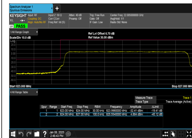
Band26(824-849)-3MHz-QPSK-26805-15RB#0-PASS
