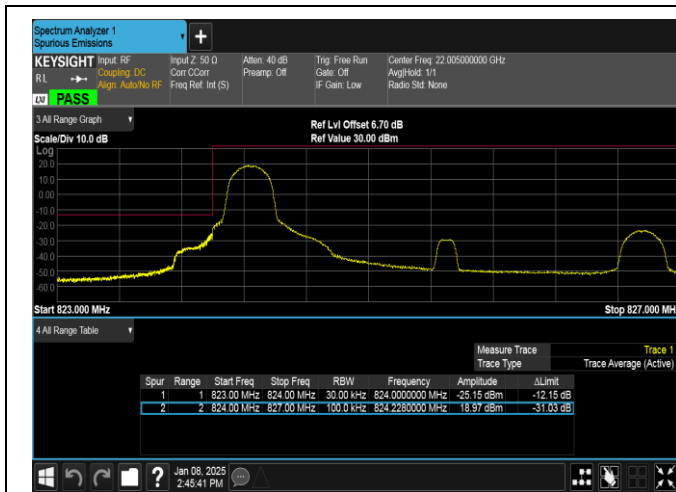
Band26(824-849)-3MHz-QPSK-26805-1RB#0-PASS
