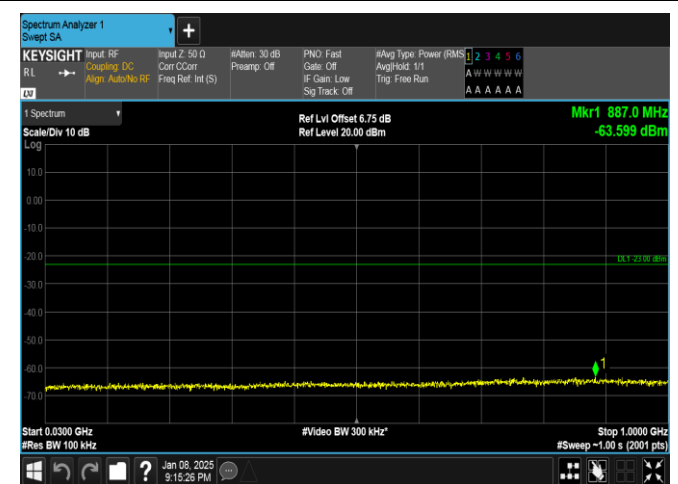
Band25-20MHz-QPSK-26365-1RB#0-30~1000-PASS
