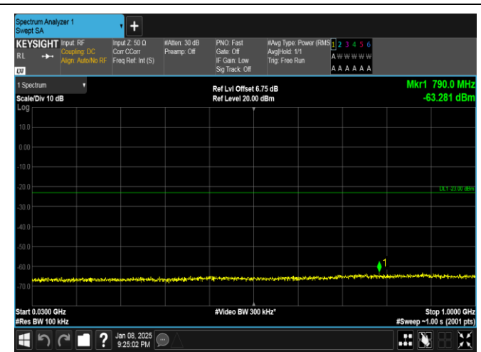
Band25-20MHz-QPSK-26590-1RB#99-30~1000-PASS
