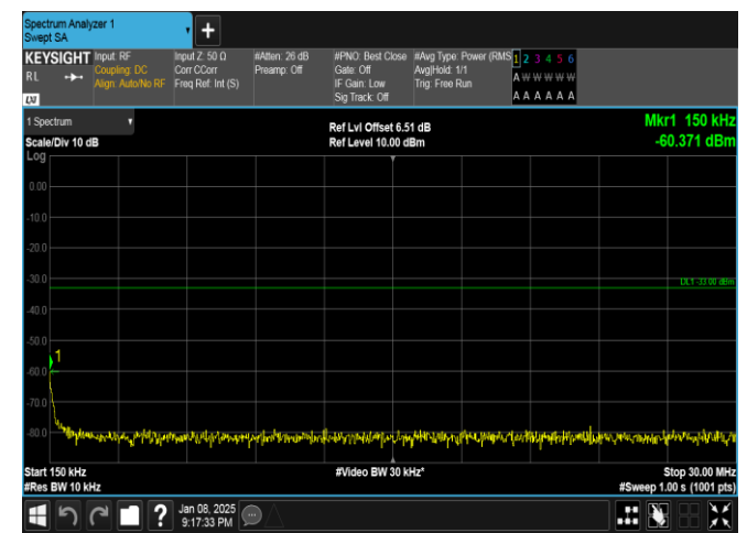
Band25-20MHz-QPSK-26365-1RB#99-0.15~30-PASS
