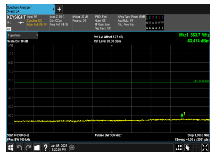
Band25-20MHz-QPSK-26365-100RB#0-30~1000-PASS
