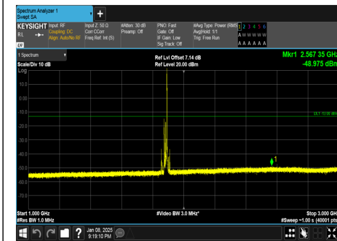
Band25-20MHz-16QAM-26365-1RB#99-1000~3000-PASS
