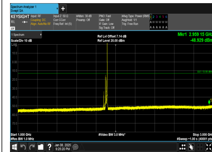
Band25-20MHz-QPSK-26590-1RB#99-1000~3000-PASS
