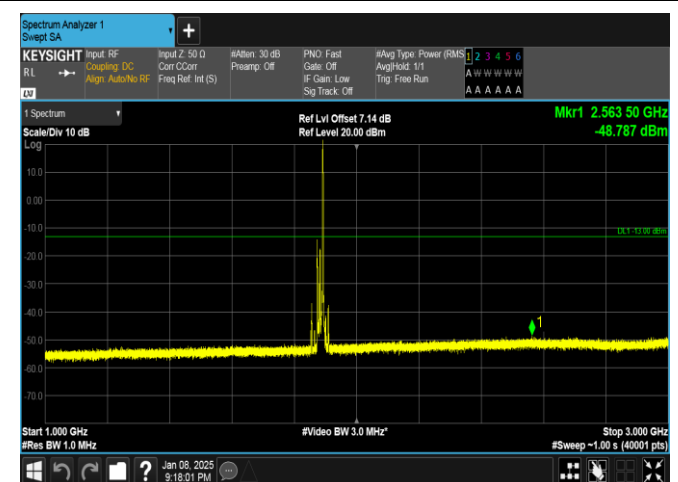
Band25-20MHz-QPSK-26365-1RB#99-1000~3000-PASS
