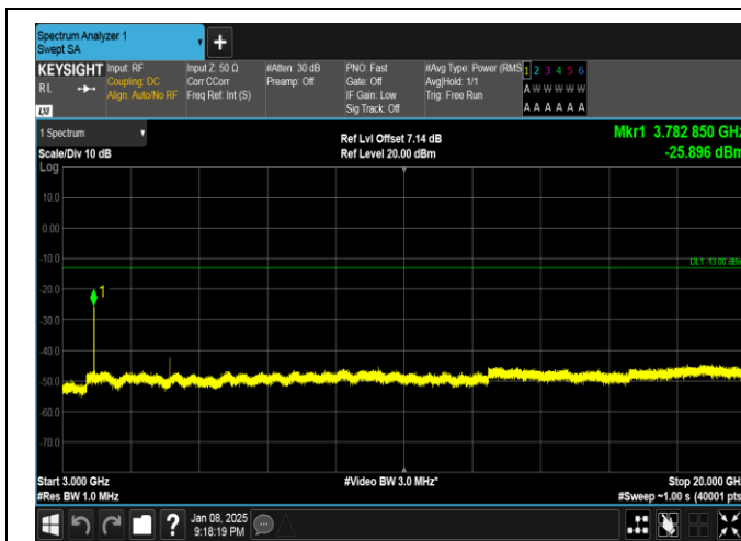
Band25-20MHz-QPSK-26365-1RB#99-3000~20000-PASS
