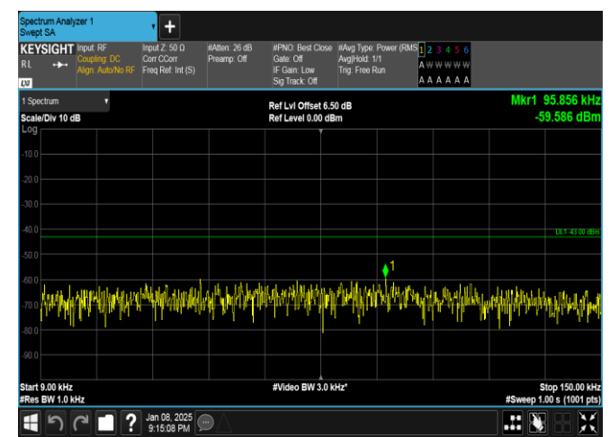
Band25-20MHz-QPSK-26365-1RB#0-0.009~0.15-PASS
