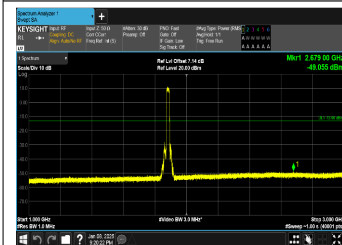
Band25-20MHz-QPSK-26365-100RB#0-1000~3000-PASS
