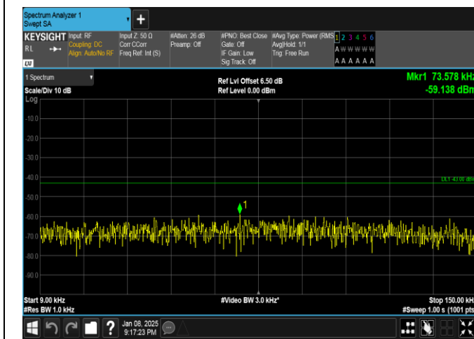
Band25-20MHz-QPSK-26365-1RB#99-0.009~0.15-PASS
