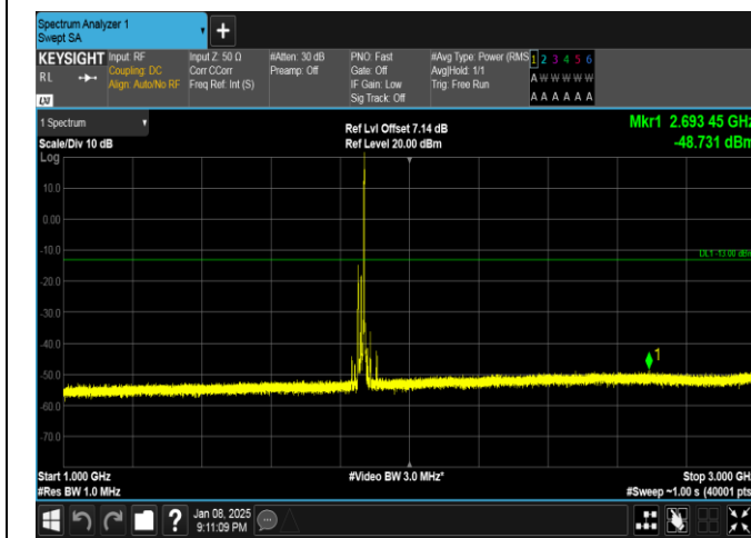
Band25-20MHz-QPSK-26140-1RB#99-1000~3000-PASS
