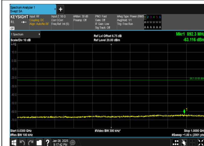
Band25-20MHz-QPSK-26365-1RB#99-30~1000-PASS
