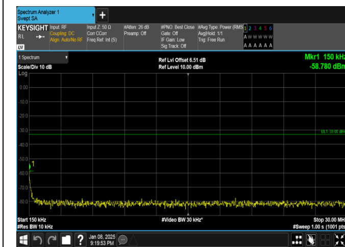
Band25-20MHz-QPSK-26365-100RB#0-0.15~30-PASS
