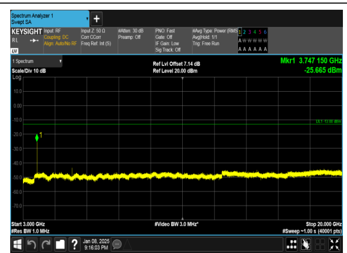
Band25-20MHz-QPSK-26365-1RB#0-3000~20000-PASS
