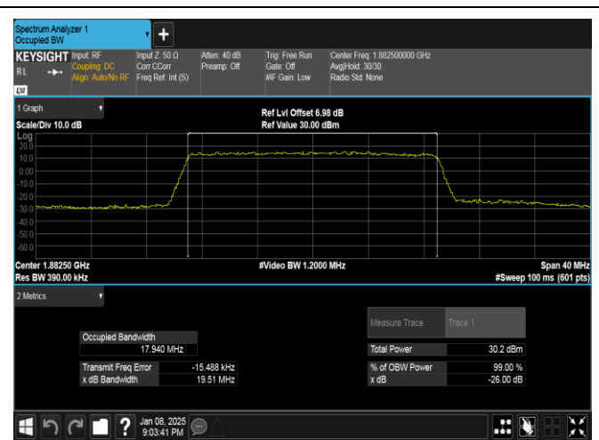
Band25-20MHz-QPSK-26365-100RB#0-PASS
