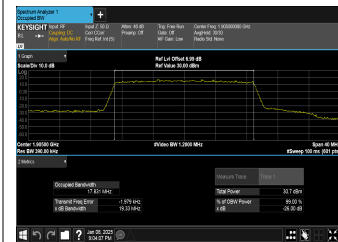
Band25-20MHz-QPSK-26590-100RB#0-PASS
