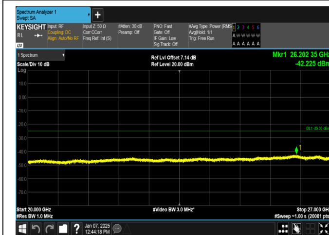
Band7-15MHz-16QAM-20825-1RB#74-20000~27000-PASS
