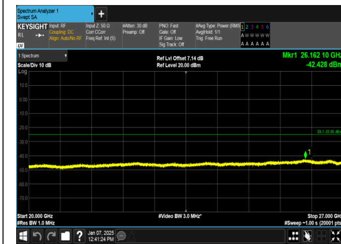
Band7-15MHz-QPSK-20825-1RB#0-20000~27000-PASS
