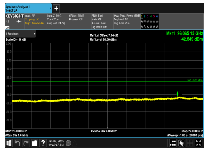
Band7-10MHz-QPSK-21100-50RB#0-20000~27000-PASS
