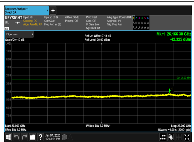
Band7-15MHz-QPSK-20825-1RB#74-20000~27000-PASS
