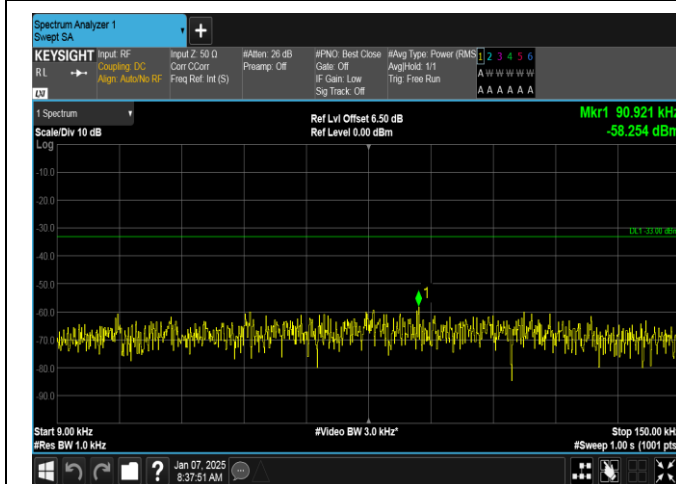
Band5-3MHz-QPSK-20635-1RB#0-0.009~0.15-PASS
