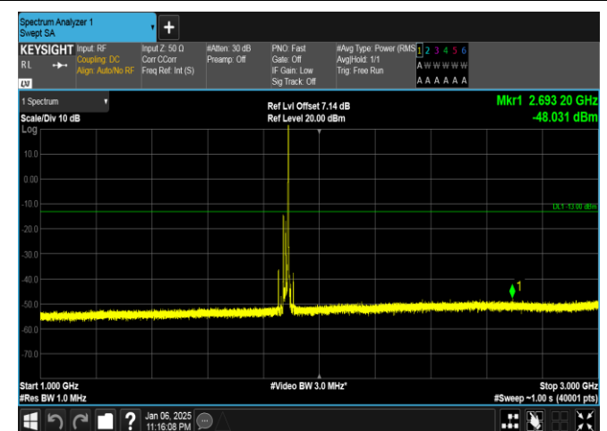
Band2-20MHz-QPSK-18900-1RB#99-1000~3000-PASS
