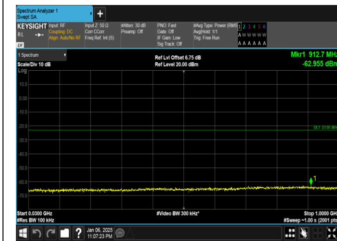
Band2-20MHz-QPSK-18700-1RB#0-30~1000-PASS
