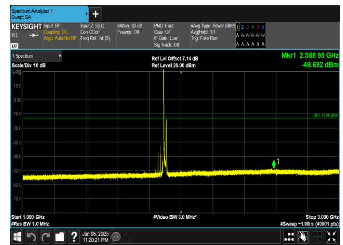
Band2-20MHz-QPSK-19100-1RB#0-1000~3000-PASS
