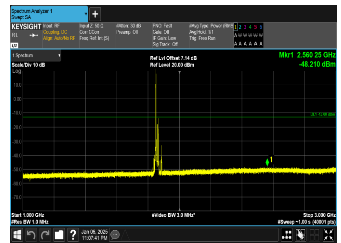
Band2-20MHz-QPSK-18700-1RB#0-1000~3000-PASS
