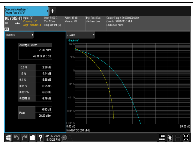
Band2-20MHz-QPSK-18700-100RB#0-PASS
