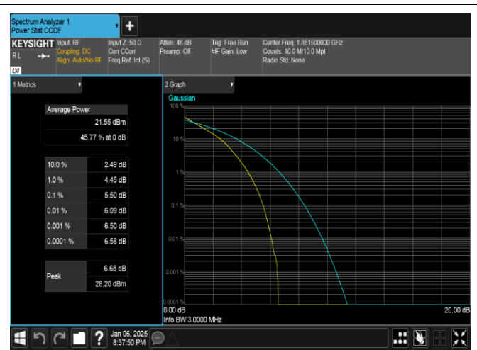
Band2-3MHz-QPSK-18615-15RB#0-PASS
