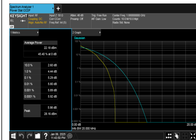
Band2-20MHz-QPSK-18900-1RB#0-PASS
