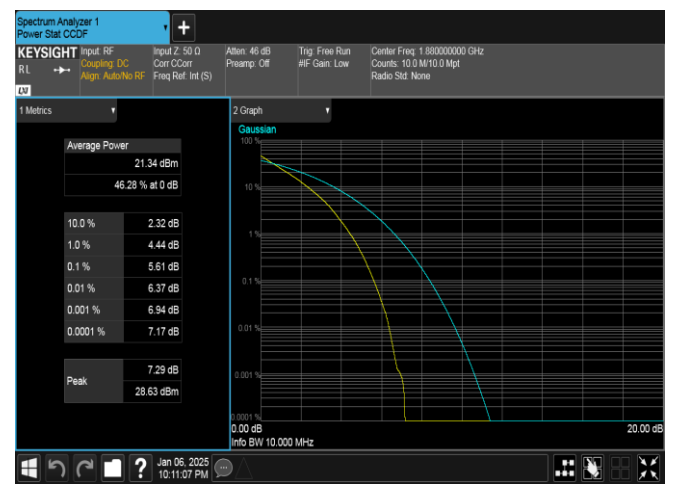
Band2-10MHz-QPSK-18900-50RB#0-PASS
