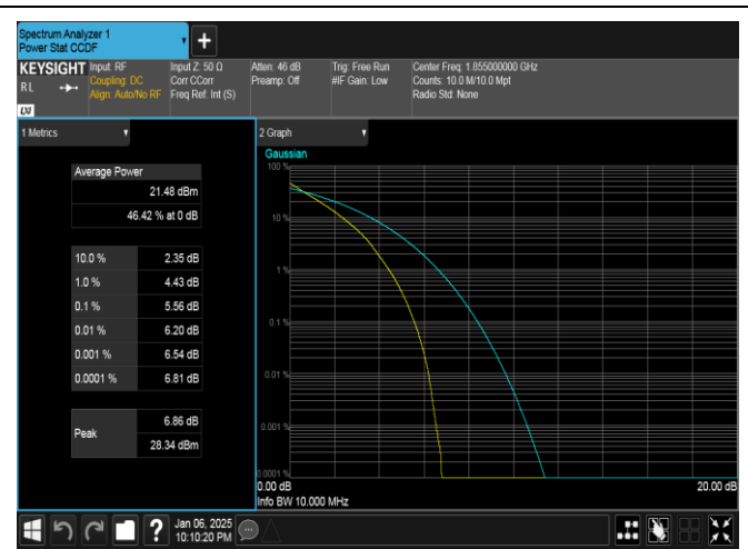
Band2-10MHz-QPSK-18650-50RB#0-PASS
