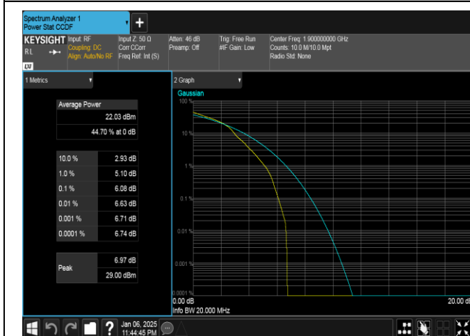
Band2-20MHz-16QAM-19100-1RB#0-PASS
