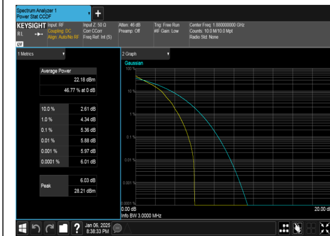
Band2-3MHz-QPSK-18900-1RB#0-PASS
