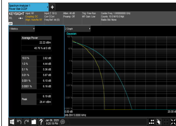
Band2-5MHz-QPSK-18900-1RB#0-PASS
