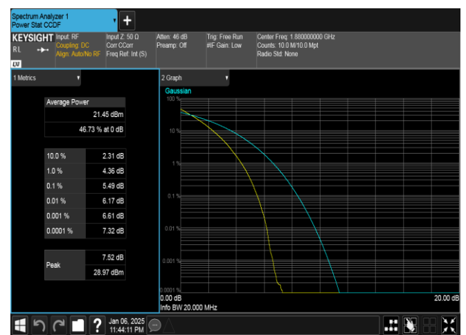
Band2-20MHz-QPSK-18900-100RB#0-PASS
