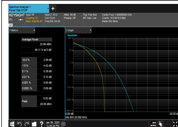
Band2-20MHz-QPSK-19100-1RB#0-PASS
