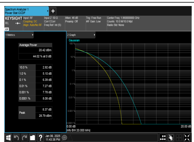
Band2-20MHz-16QAM-18700-100RB#0-PASS
