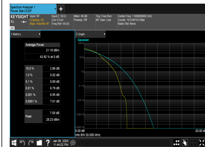
Band2-20MHz-16QAM-18900-1RB#0-PASS
