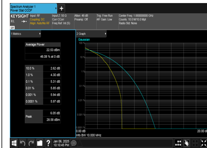
Band2-10MHz-QPSK-18900-1RB#0-PASS
