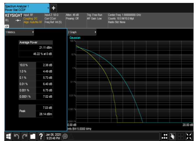
Band2-5MHz-QPSK-18900-25RB#0-PASS
