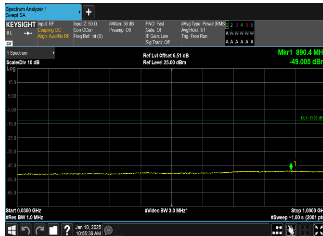
Band2-9538-2-30~1000MHz-PASS
