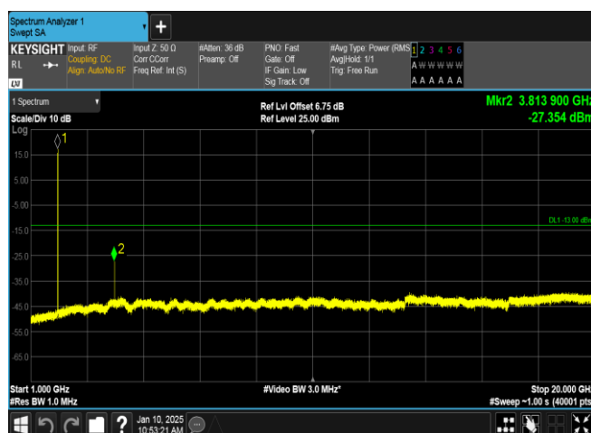
Band2-9538-1-1000~20000MHz-PASS
