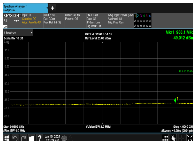
Band2-9400-1-30~1000MHz-PASS
