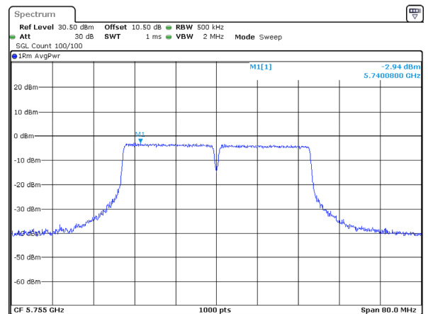
802.11ac40_5755MHz
