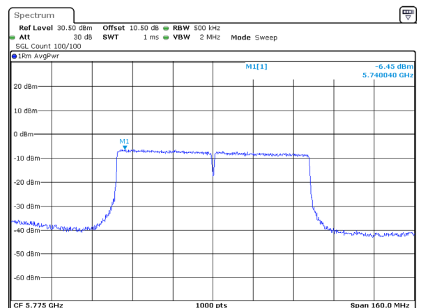
802.11ac80_5775MHz
