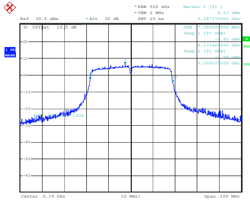
802.11ac40_5190MHz 37.500MHz
