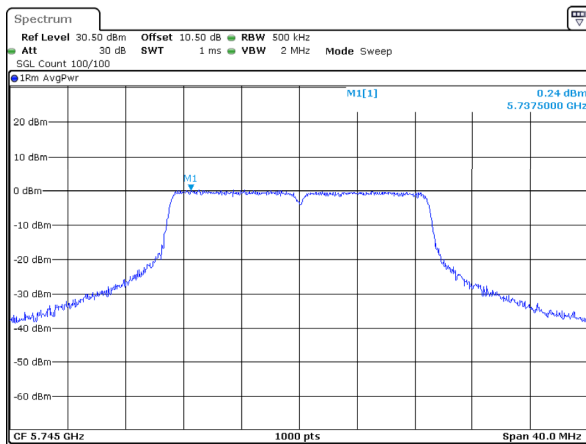
802.11ac20_5745MHz
