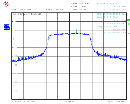
802.11ac40_5230MHz 37.750MHz
