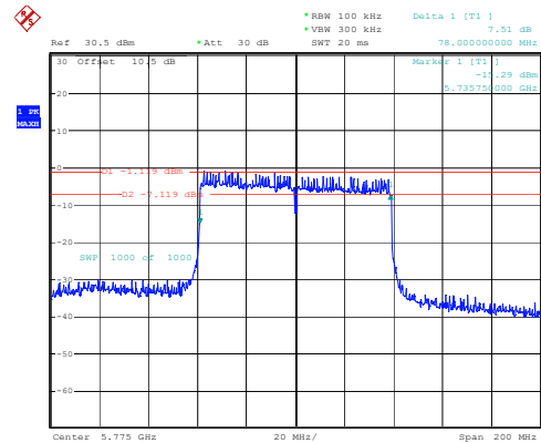
802.11ax80_5775MHz_RU_Full 78MHz
