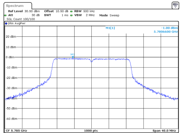
802.11ac20_5785MHz
