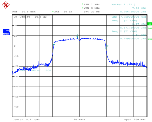
802.11ac80_5210MHz 77.750MHz
