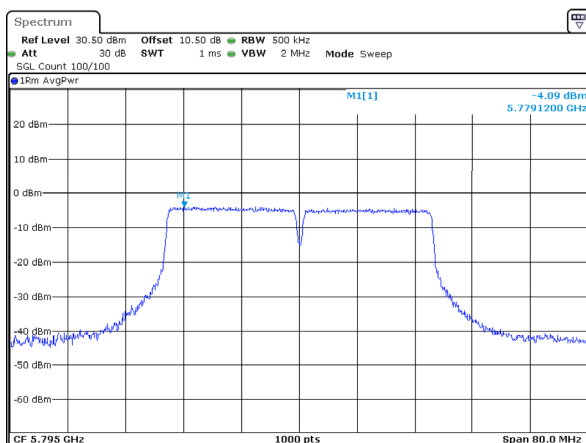
802.11ac40_5795MHz
