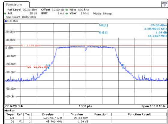
802.11ac40_5230MHz 45.746MHz
