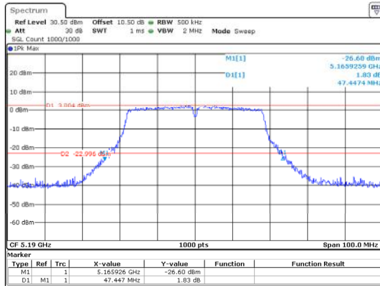
802.11ac40_5190MHz 47.447MHz
