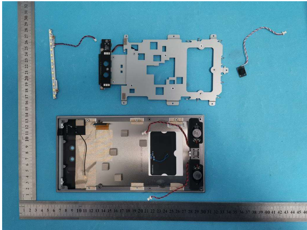
NFC ANTENNA-1
