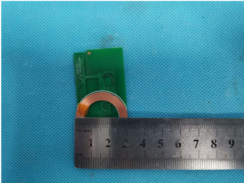
RFID ANTENNA-2
