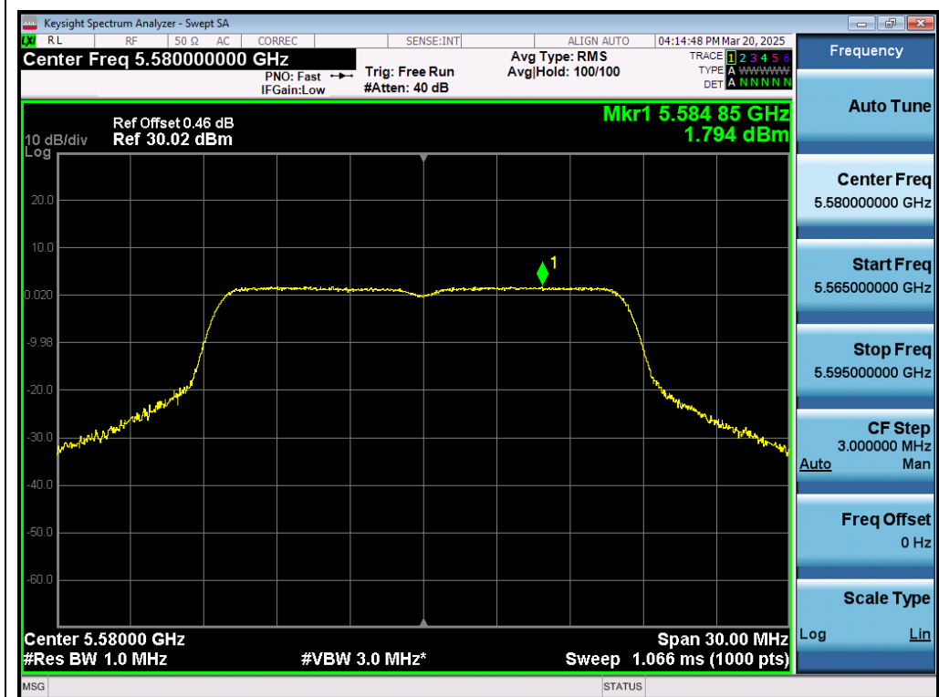
Test_Graph_802.11a_ANT1_5580_6Mbps_PSD
