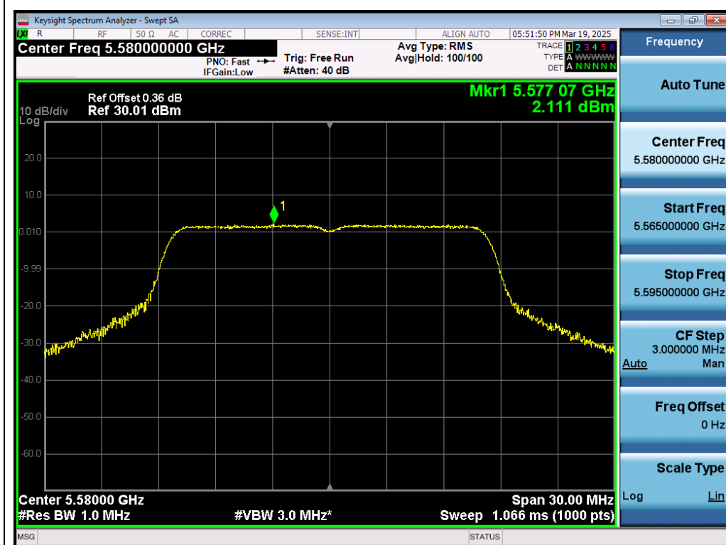
Test_Graph_802.11a_ANT1_5580_6Mbps_PSD
