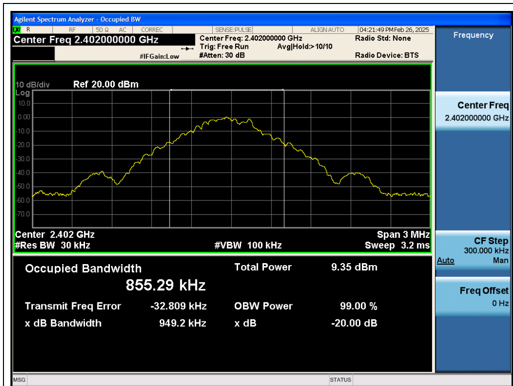
Test_Graph_BR_ANT1_2402_1Mbps_OBW
