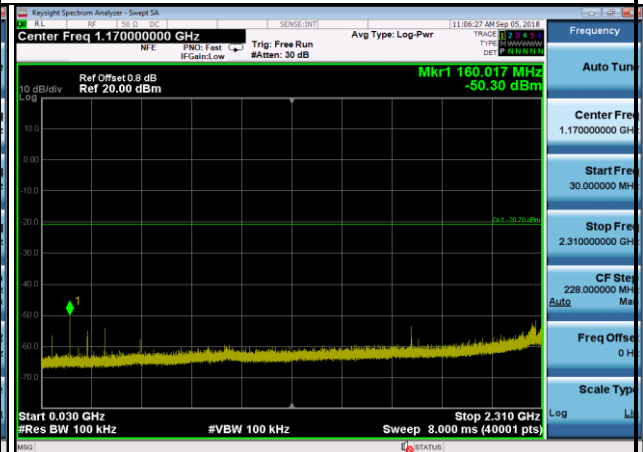
802.11g,2412MHz,Ant0,Plot 3,30MHz~2310MHz
