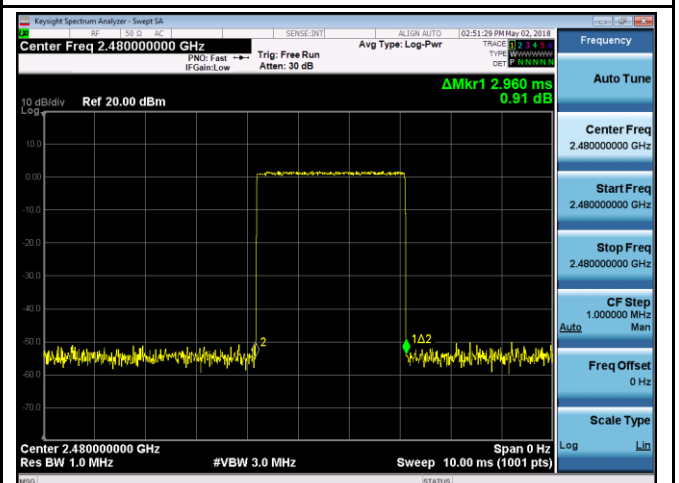
\pi/4 DQPSK - High CH 2480
