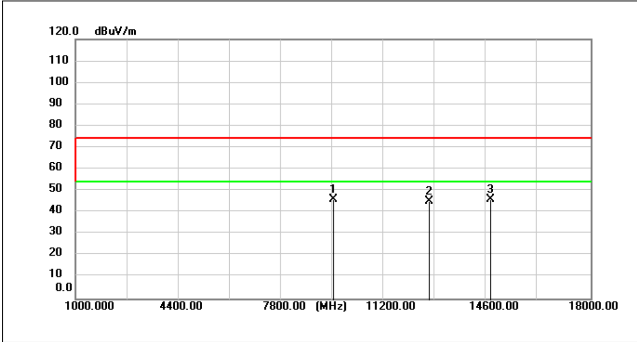
BLE_2M_TX_CH_39_Vertical
