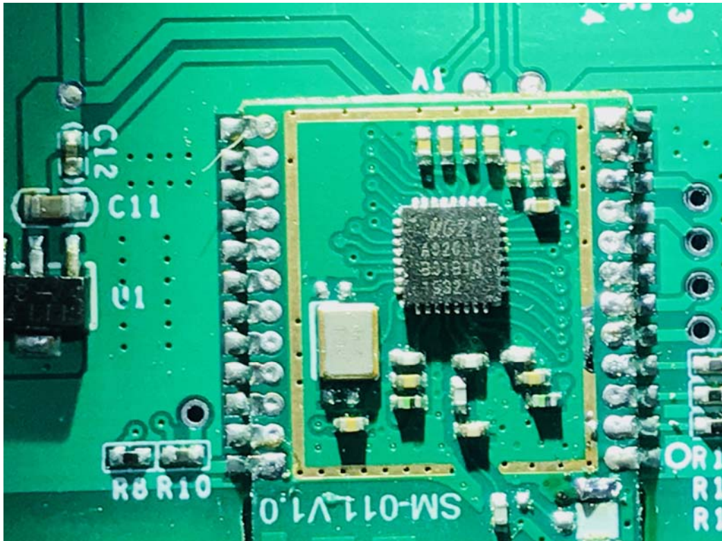
Zigbee Module
