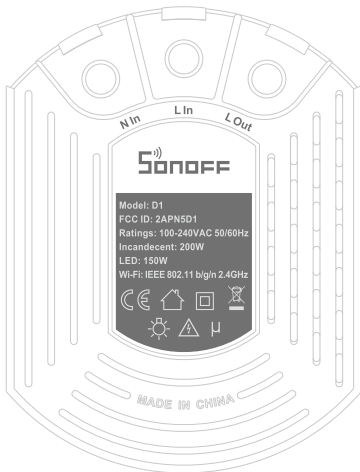
D1 调光器 丝印
