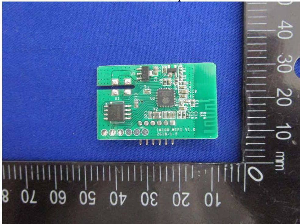
EUT –RF Module Top View
