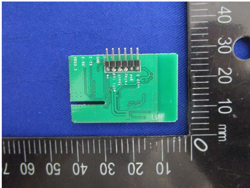
EUT –RF Module Bottom View
