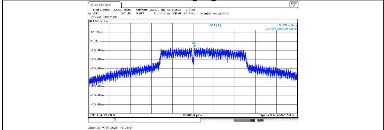
11N20SISO_Ant1_2437
