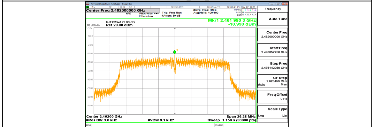
11N20SISO_Ant1_2462
