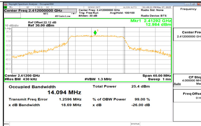
11G_Ant1_2412
