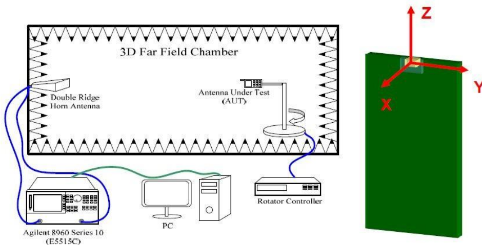
Fig.2 暗室示意图 FAR-field Chamber
