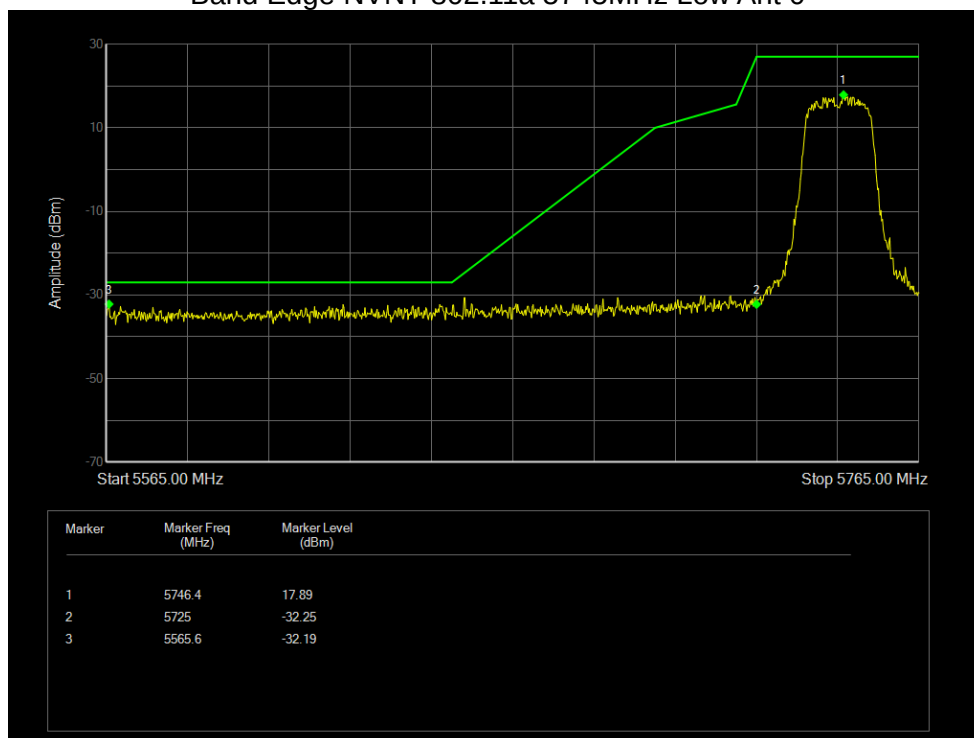
Band Edge NVNT 802.11a 5745MHz Low Ant 0
