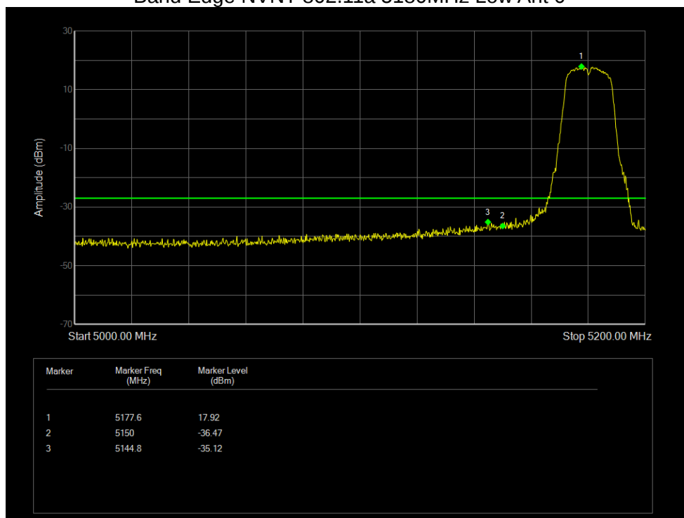
Band Edge NVNT 802.11a 5180MHz Low Ant 0
