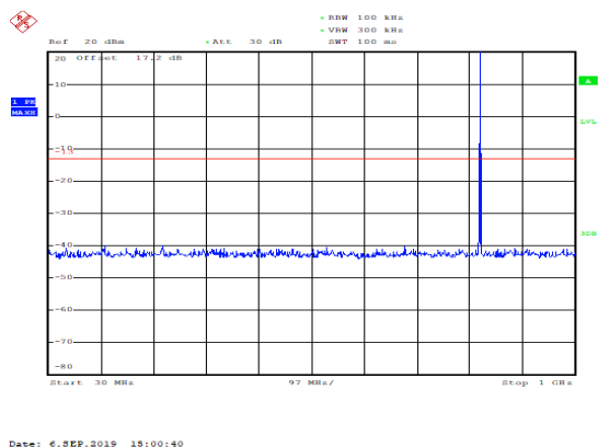
GSM 850 CH-Low 30MHz ~ 1GHz
