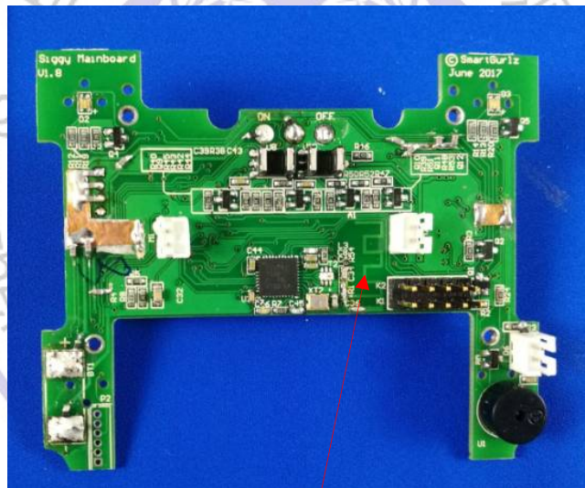
Antenna
