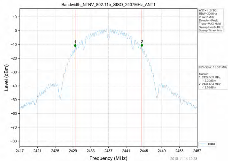
802.11b_2437MHz_SISO_ANT1
