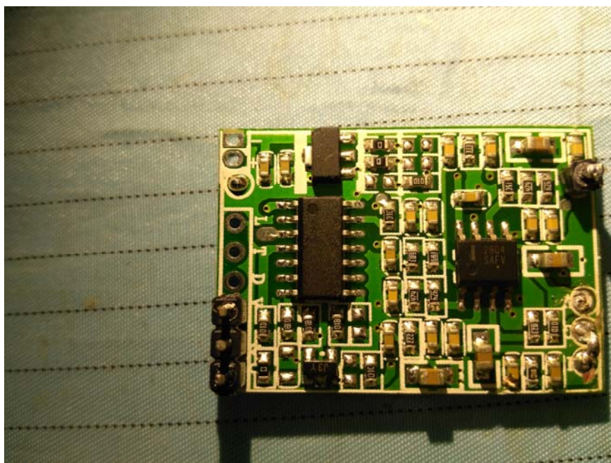
EUT – 5.8GHz Module IC Chip View
