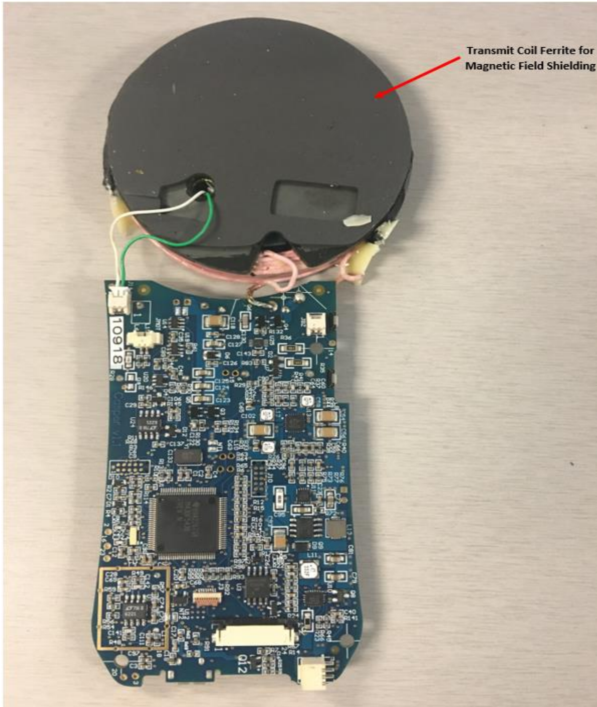
PCBA Bottom
