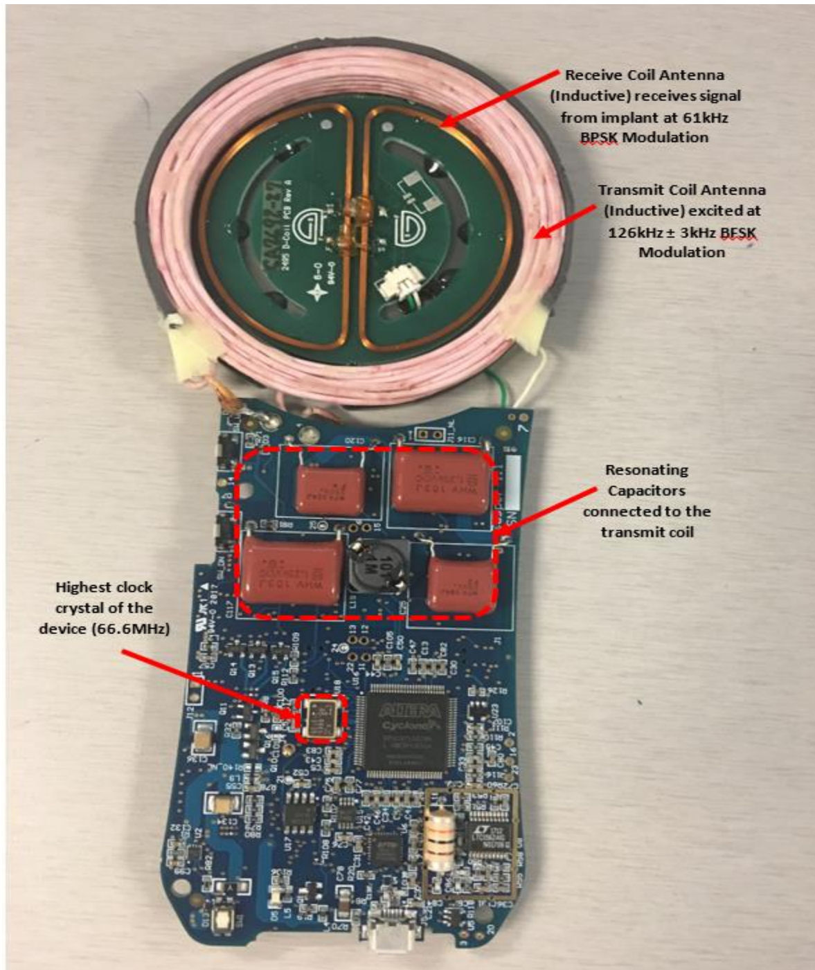
PCBA Top
