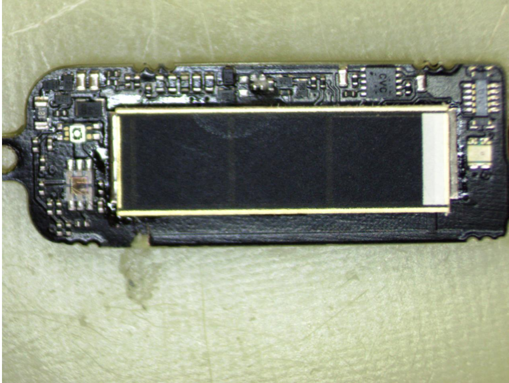
PCB bottom
