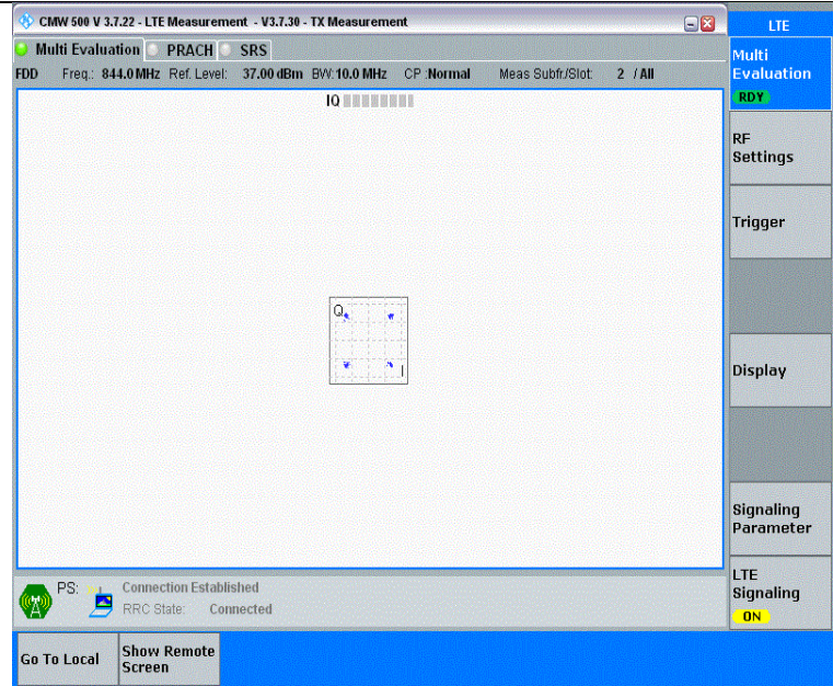
Band26(824-849)-10MHz-QPSK-26990-50RB#0-PASS
