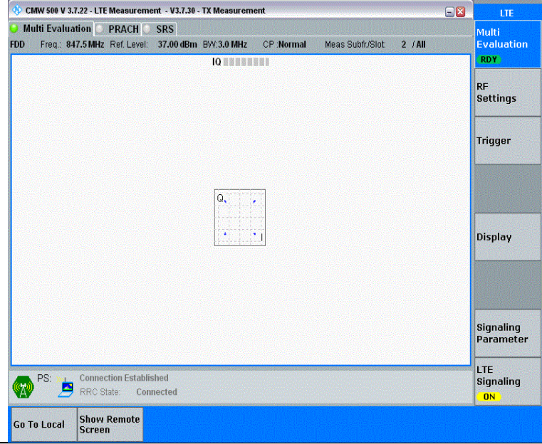
Band26(824-849)-3MHz-QPSK-27025-15RB#0-PASS
