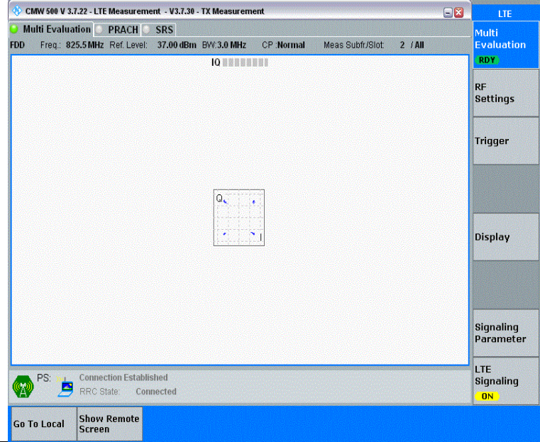
Band26(824-849)-3MHz-QPSK-26805-15RB#0-PASS
