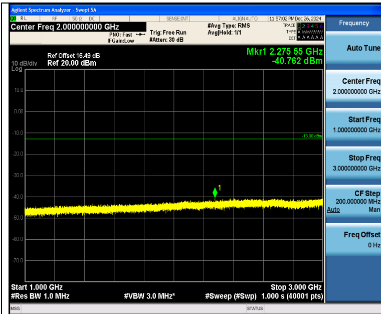
Band26 5MHz 16QAM 26815 1RB#0 1000~3000 1000~3000
