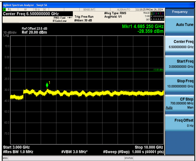
Band26 3MHz 16QAM 27025 1RB#0 3000~10000 3000~10000
