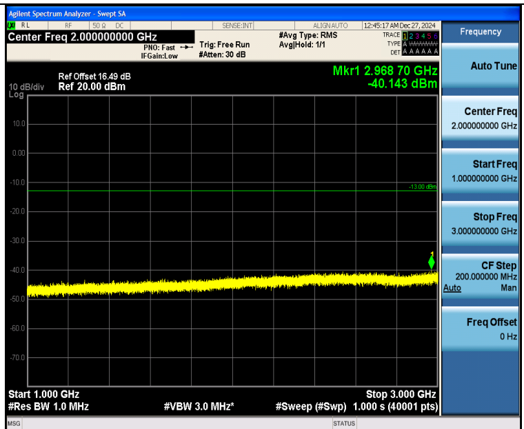
Band26 10MHz QPSK 26840 1RB#0 1000~3000 1000~3000
