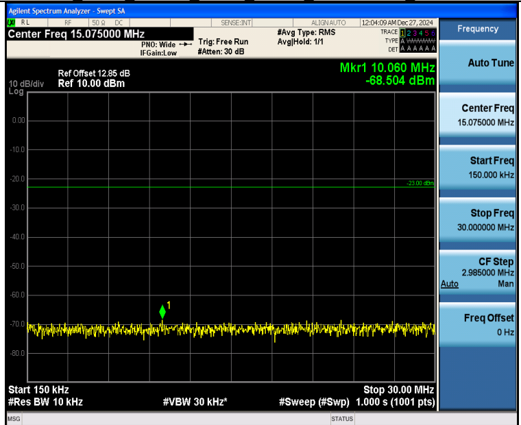
Band26 5MHz QPSK 26915 1RB#24 0.15~30 0.15~30
