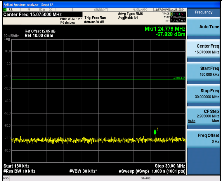
Band26 5MHz QPSK 26815 1RB#24 0.15~30 0.15~30
