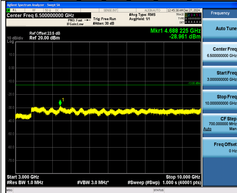
Band26 10MHz QPSK 26840 1RB#0 3000~10000 3000~10000
