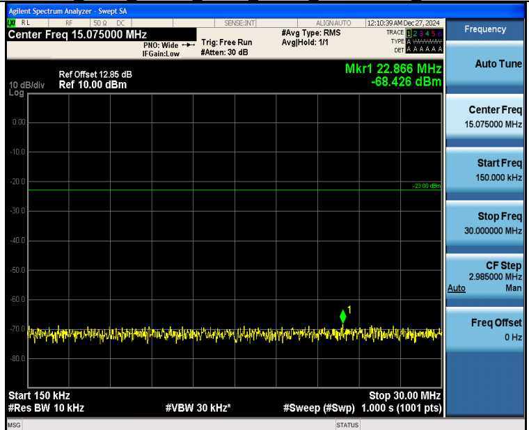
Band26 5MHz QPSK 27015 1RB#24 0.15~30 0.15~30
