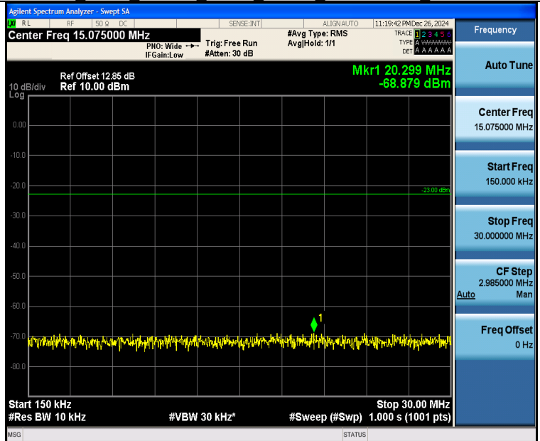
Band26 3MHz QPSK 27025 1RB#14 0.15~30 0.15~30
