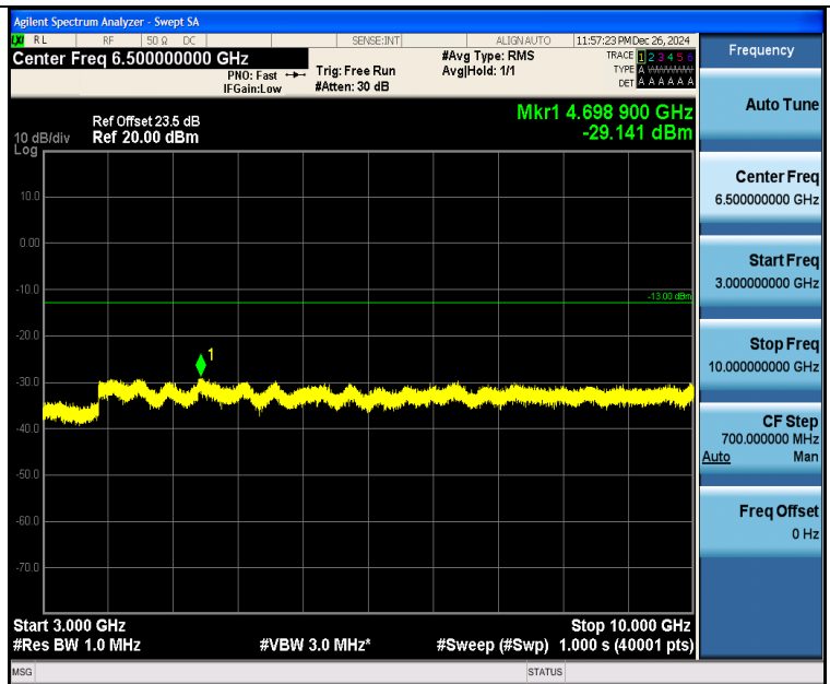
Band26 5MHz 16QAM 26815 1RB#0 3000~10000 3000~10000
