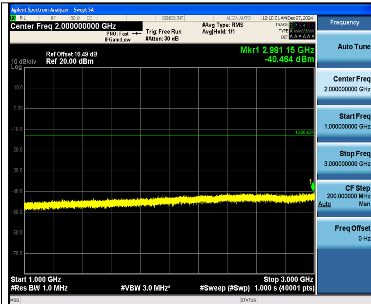
Band26 5MHz 16QAM 27015 1RB#0 1000~3000 1000~3000
