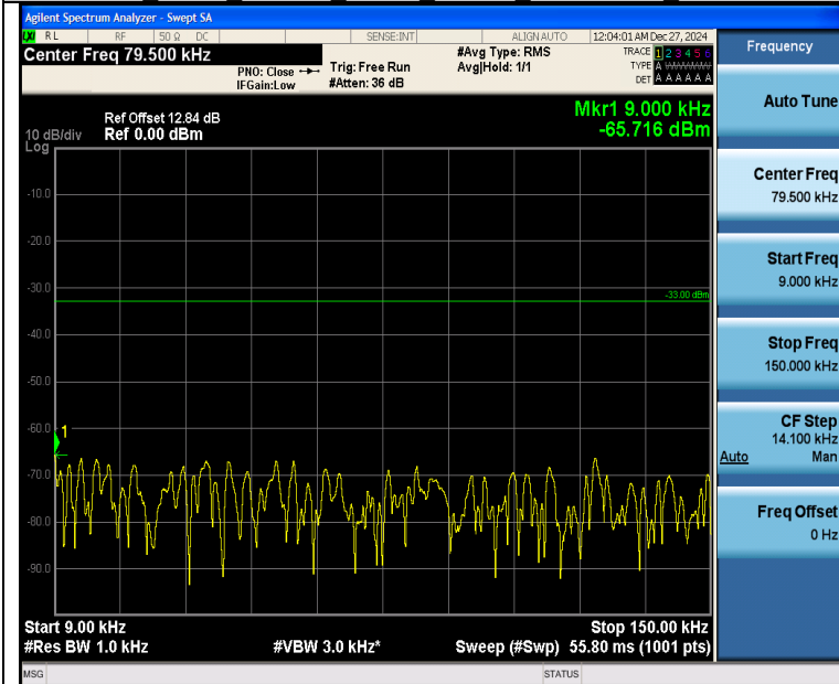
Band26 5MHz QPSK 26915 1RB#24 0.009~0.15 0.009~0.15
