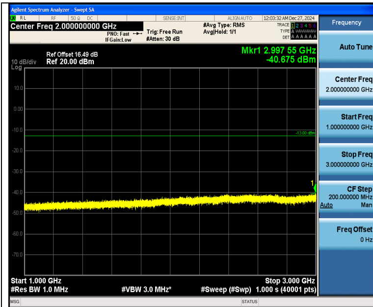
Band26 5MHz 16QAM 26915 1RB#0 1000~3000 1000~3000
