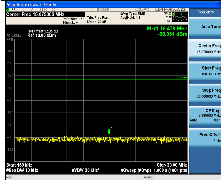
Band26 10MHz 16QAM 26840 1RB#0 0.15~30 0.15~30
