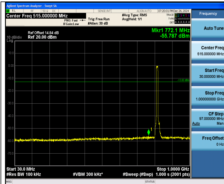
Band26 10MHz QPSK 26740 50RB#0 30~1000 30~1000
