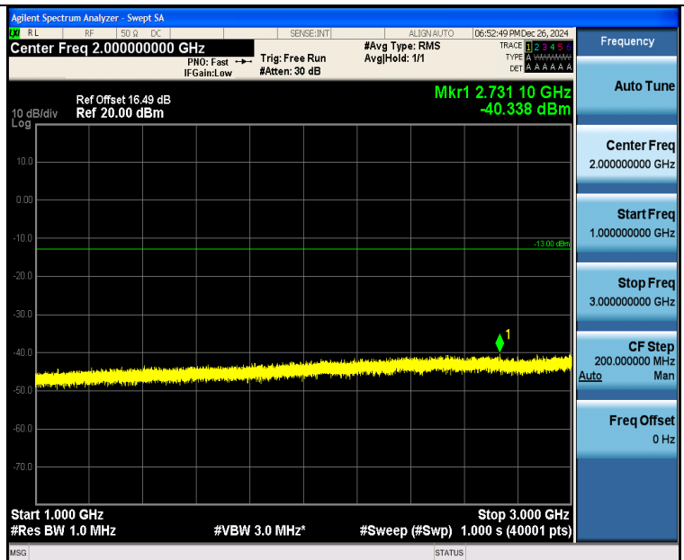
Band26 5MHz QPSK 26765 25RB#0 1000~3000 1000~3000
