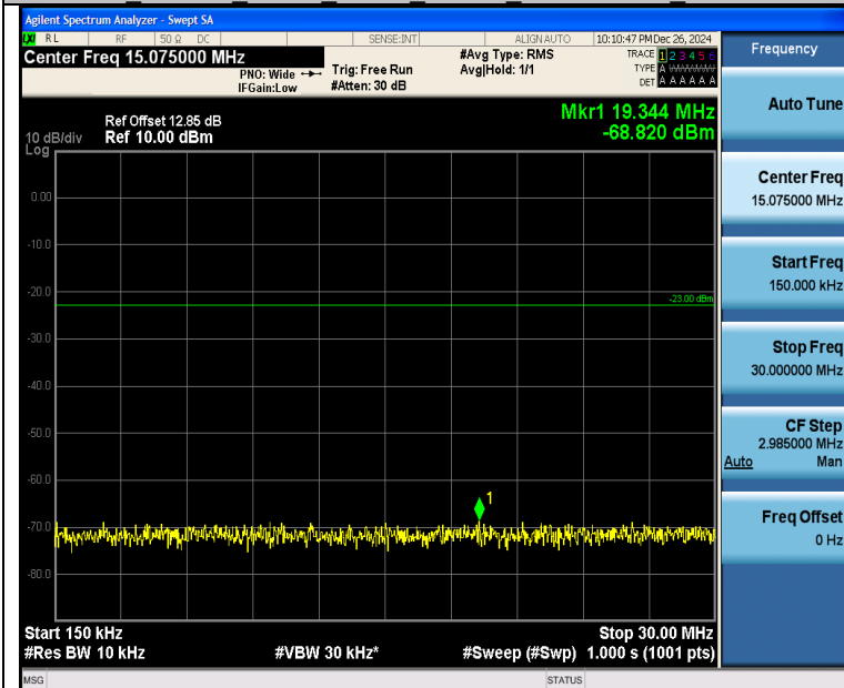
Band26 1.4MHz 16QAM 26797 1RB#0 0.15~30 0.15~30
