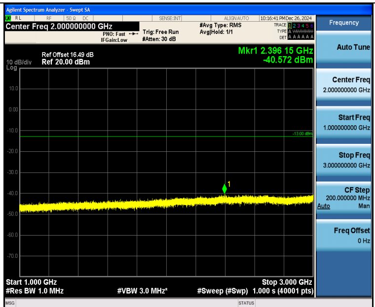
Band26 1.4MHz QPSK 26915 1RB#0 1000~3000 1000~3000
