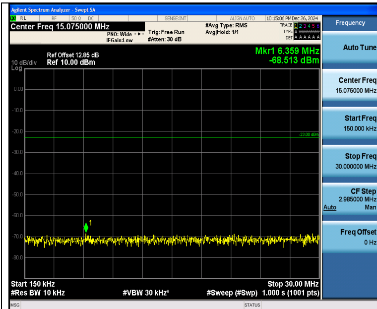
Band26 1.4MHz 16QAM 26797 6RB#0 0.15~30 0.15~30
