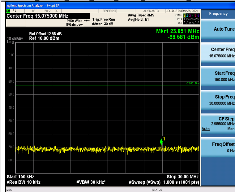
Band26 1.4MHz 16QAM 26915 1RB#0 0.15~30 0.15~30
