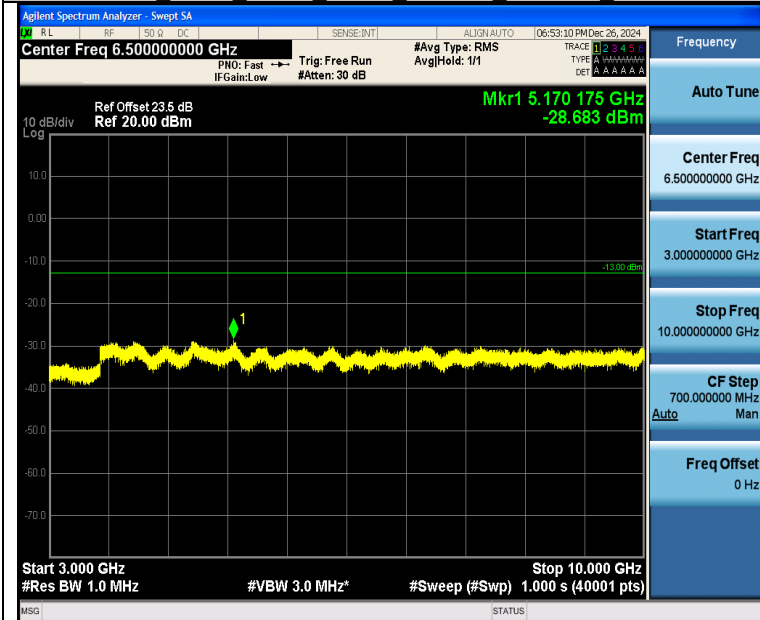
Band26 5MHz QPSK 26765 25RB#0 3000~10000 3000~10000
