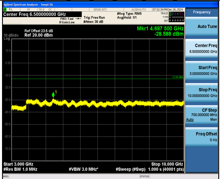
Band26 15MHz QPSK 26765 75RB#0 3000~10000 3000~10000
