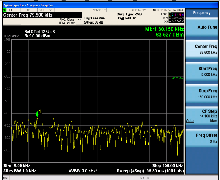
Band26 1.4MHz 16QAM 26915 1RB#0 0.009~0.15 0.009~0.15
