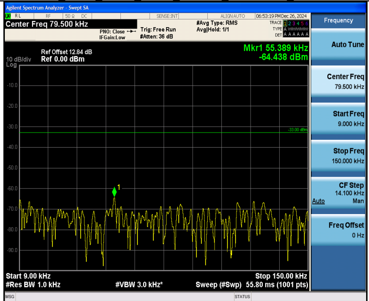
Band26 5MHz 16QAM 26765 25RB#0 0.009~0.15 0.009~0.15
