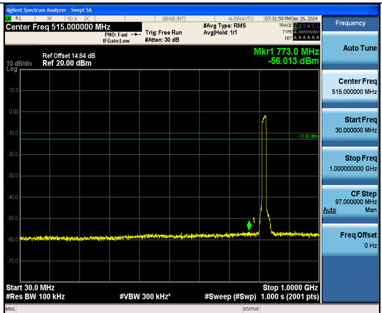
Band26 15MHz QPSK 26765 75RB#0 30~1000 30~1000
