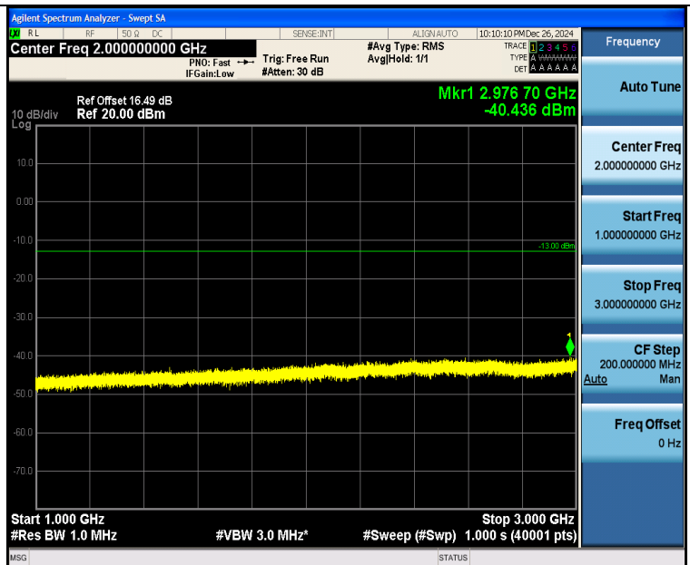
Band26 1.4MHz QPSK 26797 1RB#0 1000~3000 1000~3000
