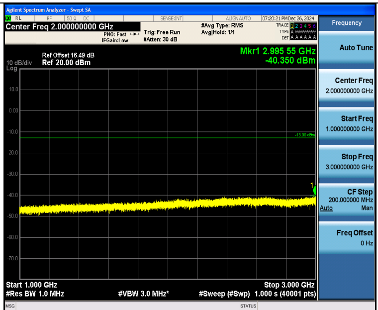
Band26 10MHz QPSK 26740 50RB#0 1000~3000 1000~3000
