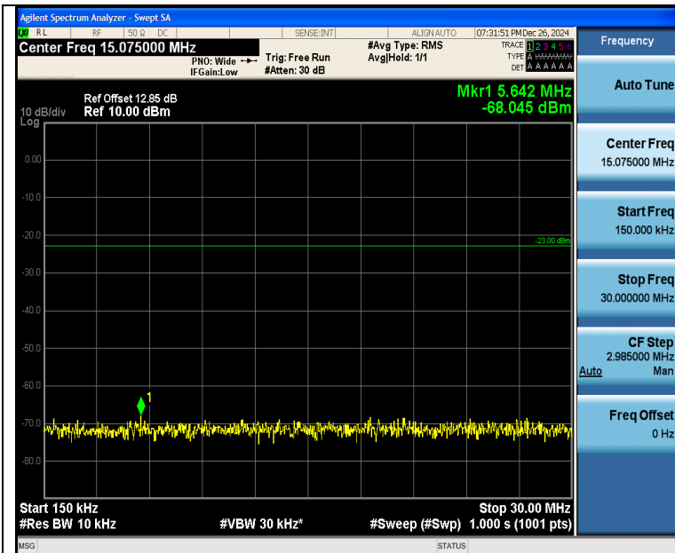
Band26 15MHz QPSK 26765 75RB#0 0.15~30 0.15~30
