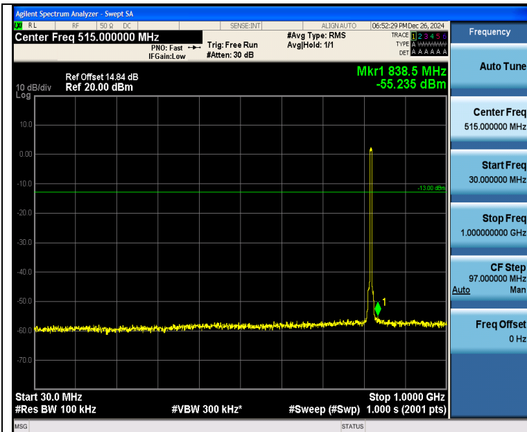
Band26 5MHz QPSK 26765 25RB#0 30~1000 30~1000
