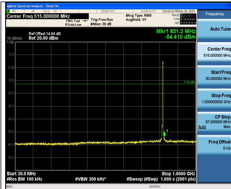
Band26 3MHz QPSK 26775 15RB#0 30~1000 30~1000
