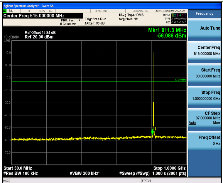
Band26 3MHz 16QAM 26740 1RB#14 30~1000 30~1000
