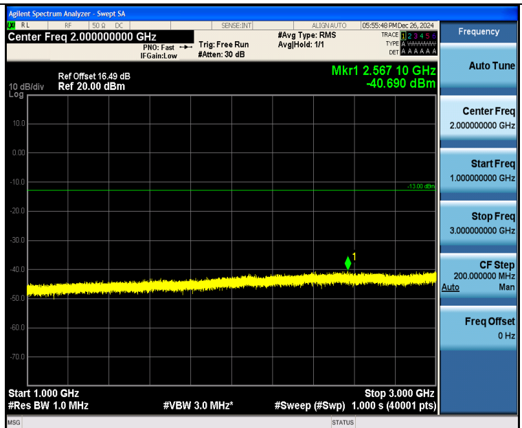
Band26 3MHz QPSK 26740 15RB#0 1000~3000 1000~3000
