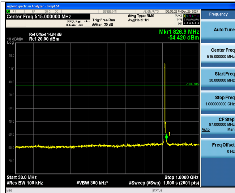
Band26 3MHz QPSK 26740 15RB#0 30~1000 30~1000
