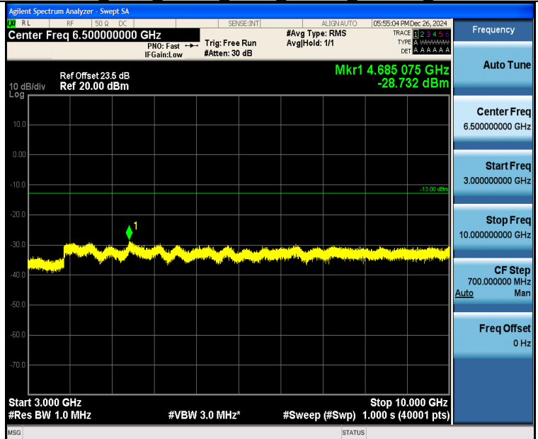
Band26 3MHz 16QAM 26740 1RB#14 3000~10000 3000~10000
