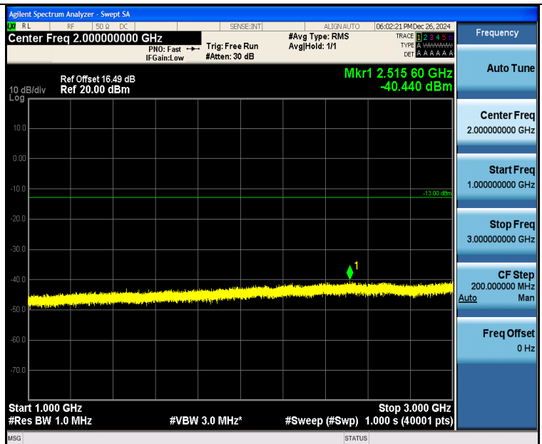
Band26 3MHz QPSK 26775 15RB#0 1000~3000 1000~3000
