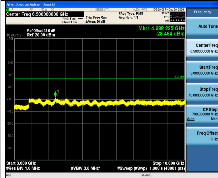
Band26 3MHz QPSK 26740 15RB#0 3000~10000 3000~10000
