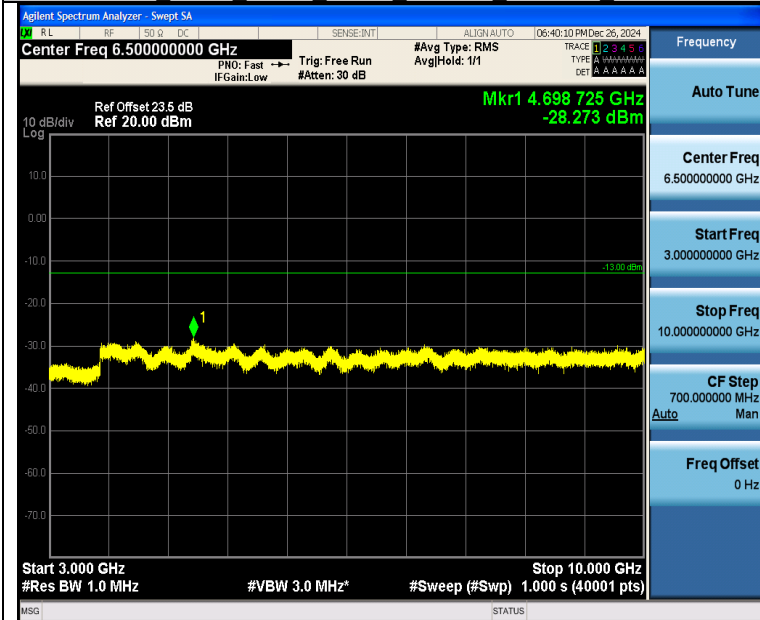
Band26 5MHz QPSK 26715 25RB#0 3000~10000 3000~10000
