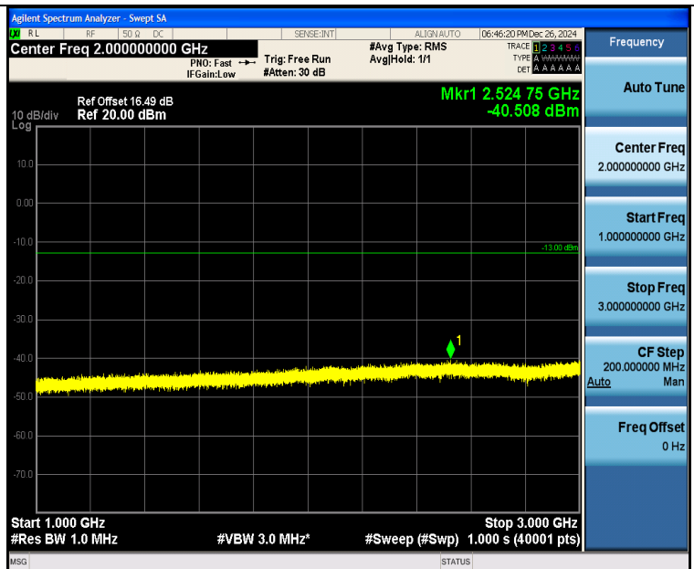
Band26 5MHz QPSK 26740 25RB#0 1000~3000 1000~3000
