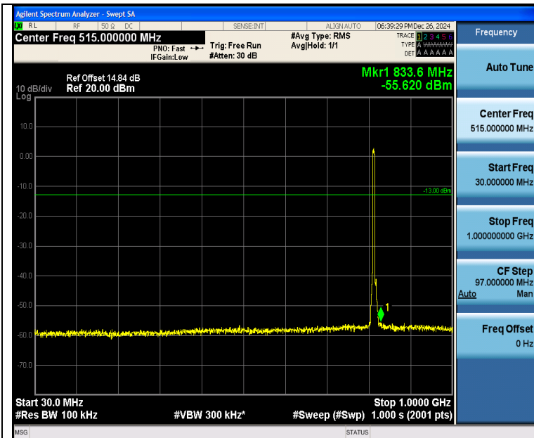
Band26 5MHz QPSK 26715 25RB#0 30~1000 30~1000
