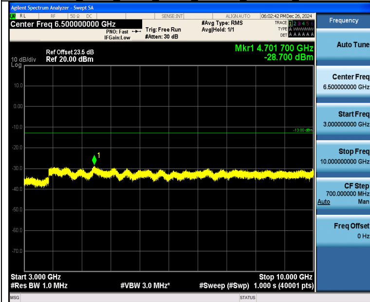
Band26 3MHz QPSK 26775 15RB#0 3000~10000 3000~10000
