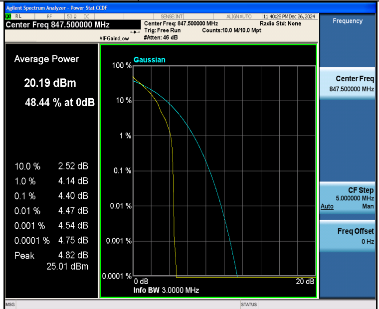
Band26(824-849)-3MHz-QPSK-27025-1RB#0-PASS
