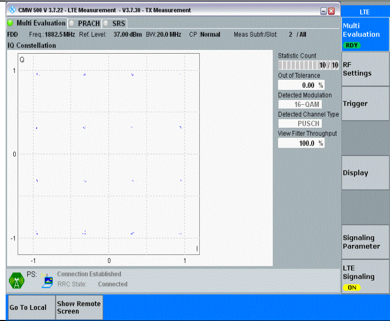
Band25-20MHz-16QAM-26365-1RB#0-PASS
