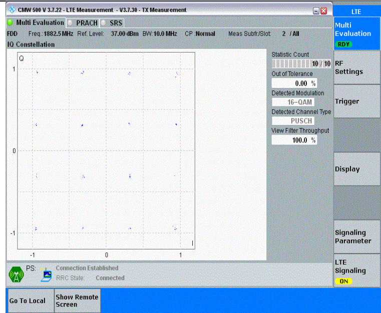
Band25-10MHz-16QAM-26365-1RB#0-PASS
