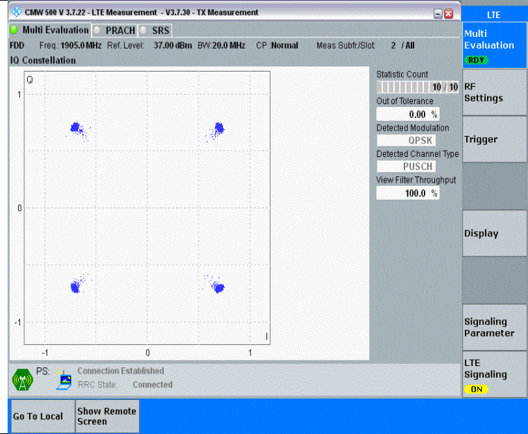
Band25-20MHz-QPSK-26590-100RB#0-PASS
