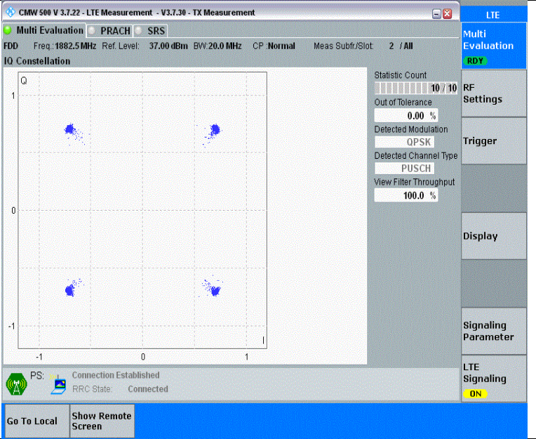
Band25-20MHz-QPSK-26365-100RB#0-PASS
