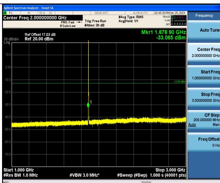
Band25 1.4MHz QPSK 26365 1RB#0 1000~3000 1000~3000
