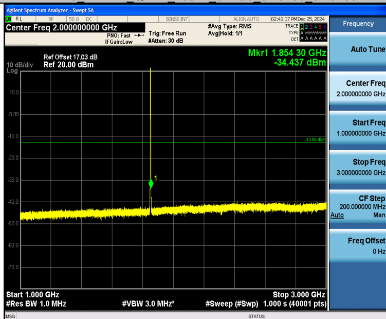
Band25 1.4MHz QPSK 26047 6RB#0 1000~3000 1000~3000
