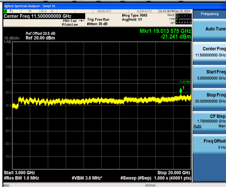
Band25 1.4MHz QPSK 26047 6RB#0 3000~20000 3000~20000
