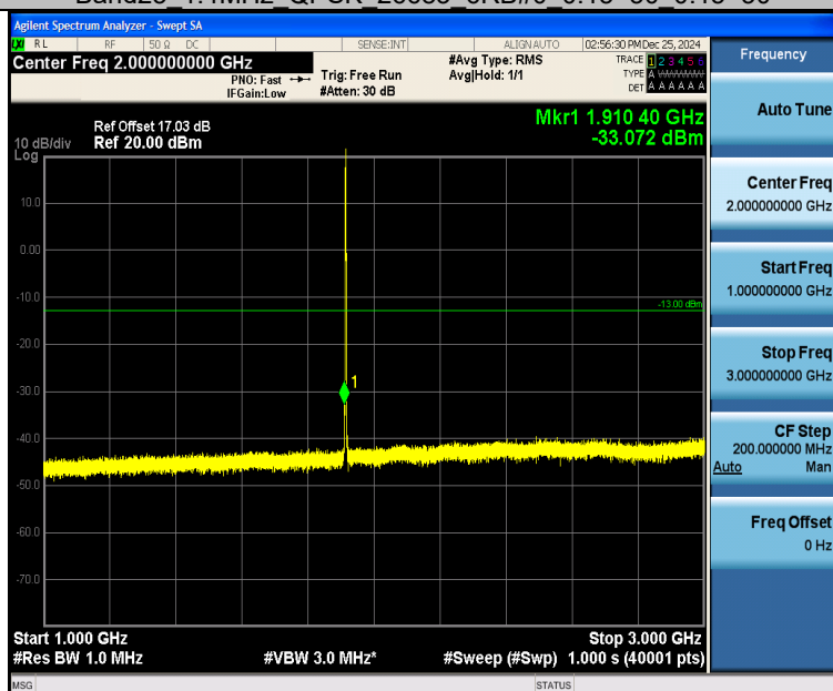
Band25 1.4MHz QPSK 26683 6RB#0 1000~3000 1000~3000
