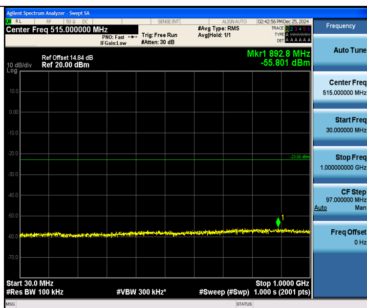
Band25 1.4MHz QPSK 26047 6RB#0 30~1000 30~1000
