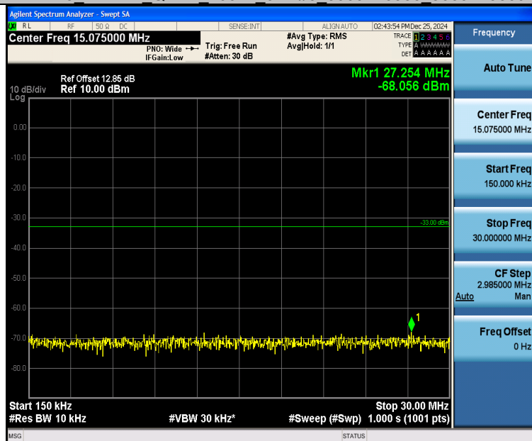
Band25 1.4MHz 16QAM 26047 6RB#0 0.15~30 0.15~30
