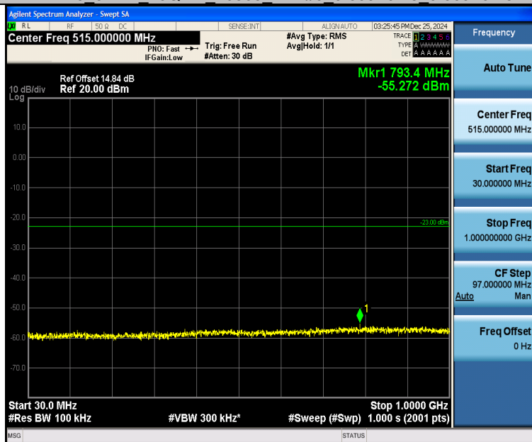
Band25 3MHz 16QAM 26365 1RB#0 30~1000 30~1000
