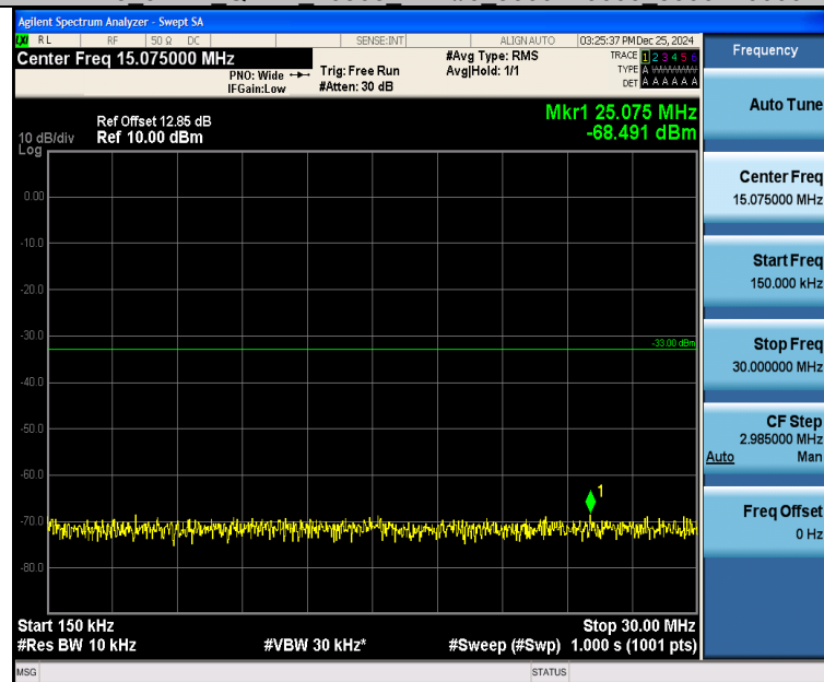
Band25 3MHz 16QAM 26365 1RB#0 0.15~30 0.15~30
