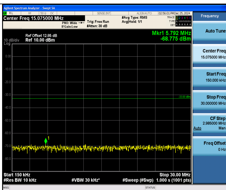
Band25 1.4MHz QPSK 26683 6RB#0 0.15~30 0.15~30
