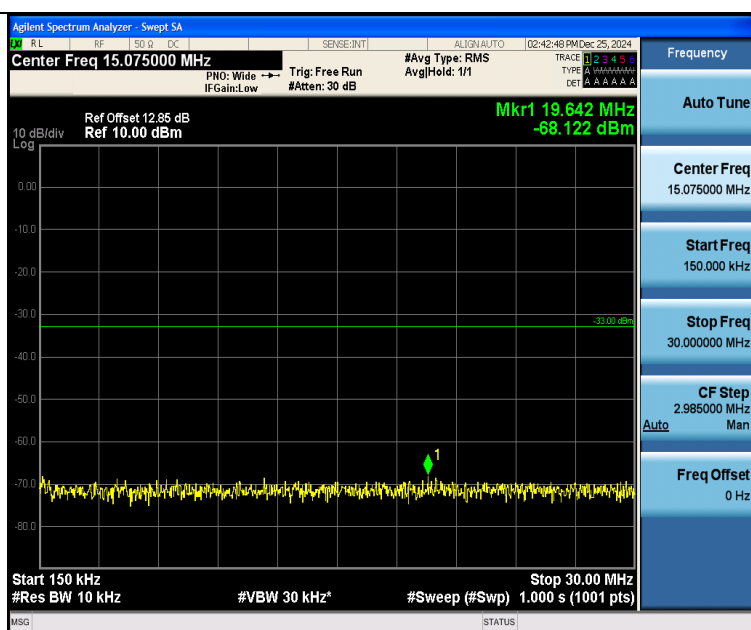
Band25 1.4MHz QPSK 26047 6RB#0 0.15~30 0.15~30
