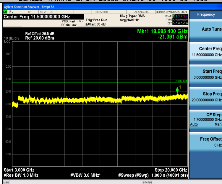
Band25 1.4MHz QPSK 26683 6RB#0 3000~20000 3000~20000
