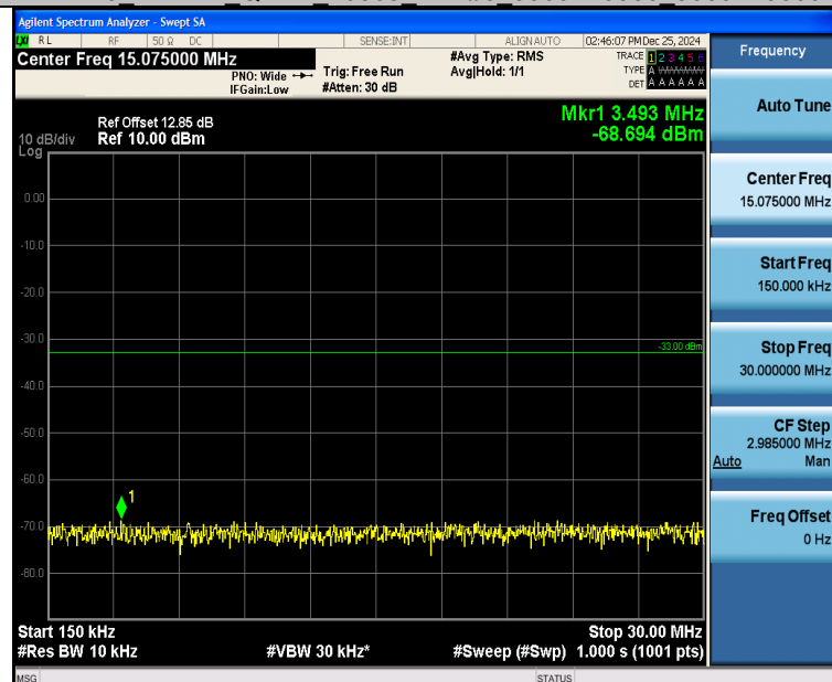
Band25 1.4MHz 16QAM 26365 1RB#0 0.15~30 0.15~30
