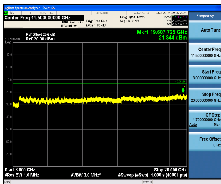
Band25 3MHz QPSK 26365 1RB#0 3000~20000 3000~20000
