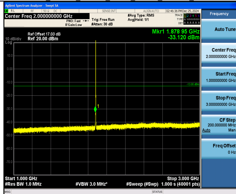
Band25 1.4MHz 16QAM 26365 1RB#0 1000~3000 1000~3000
