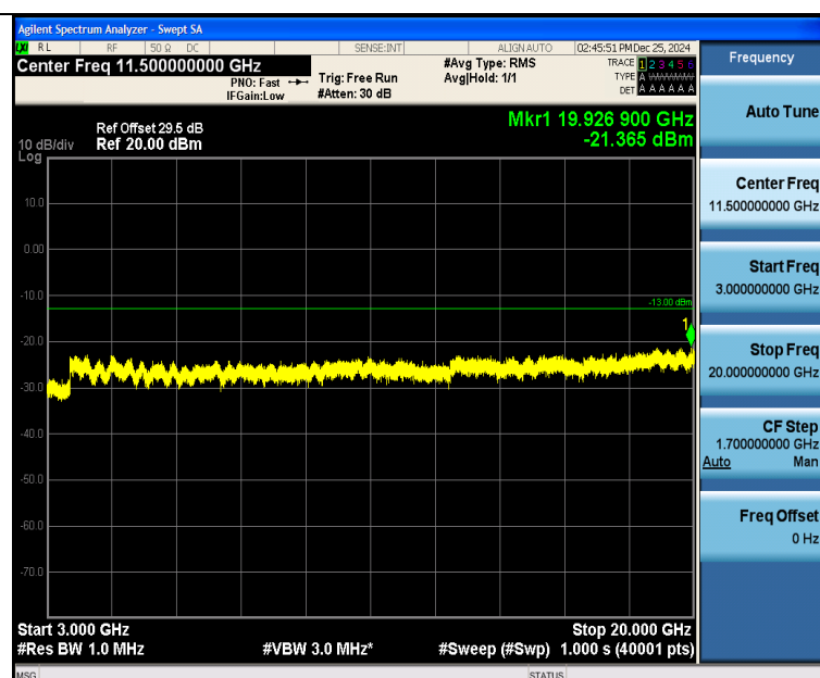
Band25 1.4MHz QPSK 26365 1RB#0 3000~20000 3000~20000
