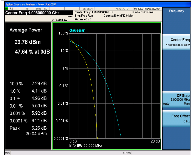
Band25-20MHz-QPSK-26590-100RB#0-PASS
