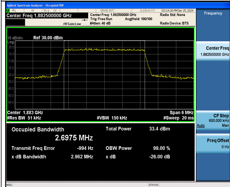
Band25-3MHz-QPSK-26365-15RB#0-PASS
