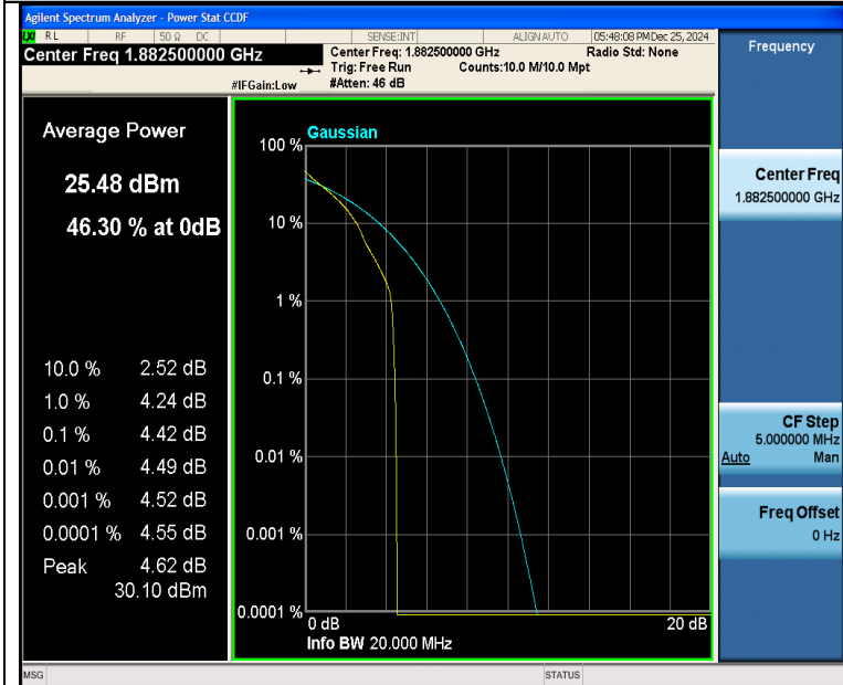
Band25-20MHz-QPSK-26365-1RB#0-PASS
