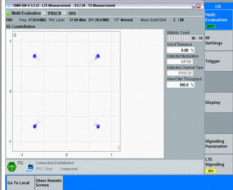
Band4-20MHz-QPSK-20050-100RB#0-PASS
