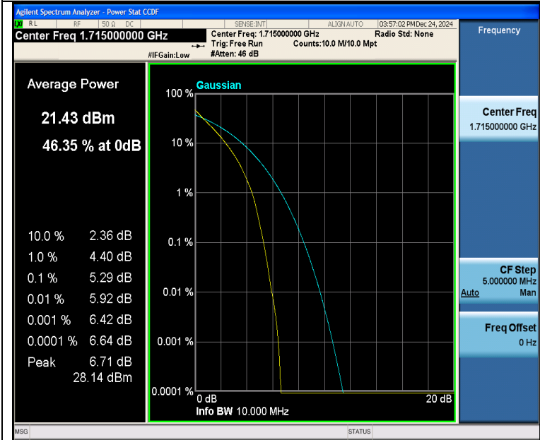
Band4-10MHz-QPSK-20000-50RB#0-PASS
