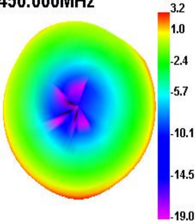
2450.000MHz
