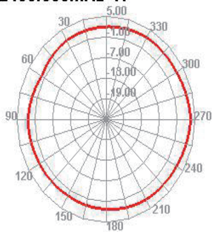
2480.000MHz H
