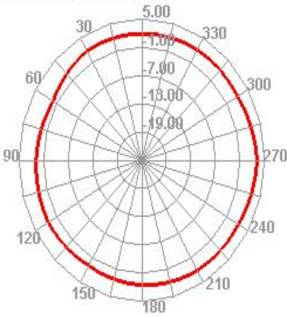
2450.000MHz H
