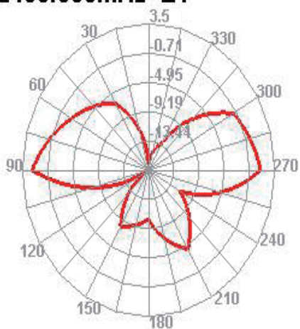
2480.000MHz E1
