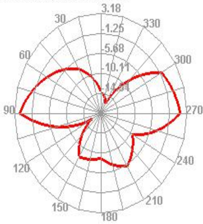
2450.000MHz E1
