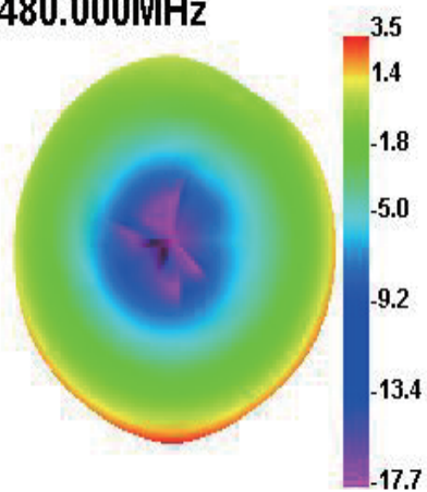
2480.000MHz
