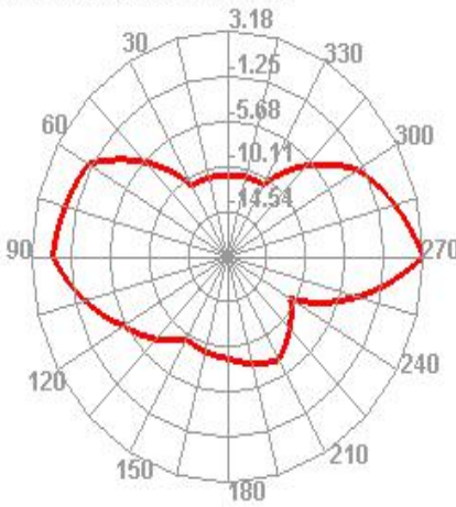
2450.000MHz E2
