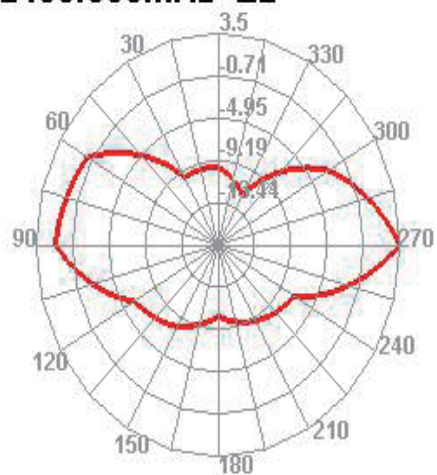
2480.000MHz E2
