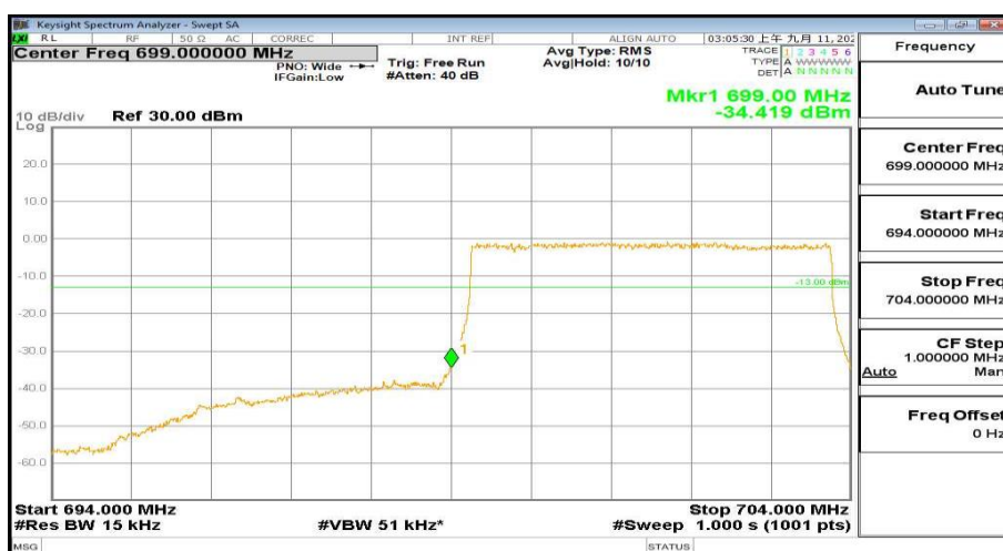
694MHz-704MHz_FreqLow_BW(5MHz)_RB(25@0)_QPSK_Band12
