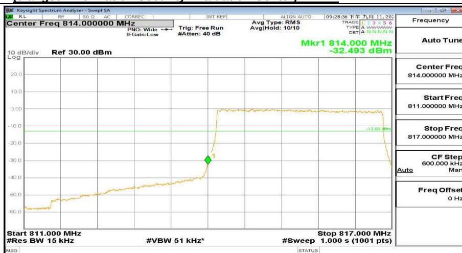
811MHz-817MHz_FreqLow_BW(_3MHz)_RB(15@0)_QPSK_Band26
