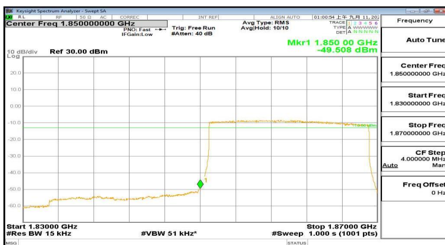
1830MHz-1870MHz_FreqLow_BW( 20MHz)_RB(100@0)_QPSK_Band25
