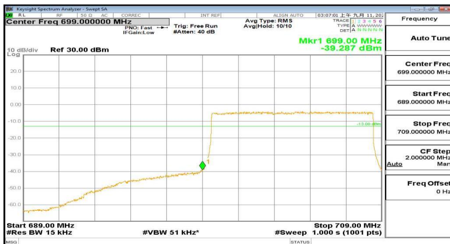
689MHz-709MHz_FreqLow_BW(10MHz)_RB(50@0)_QPSK_Band12
