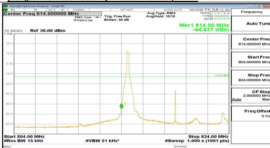
804MHz-824MHz_FreqLow_BW(10MHz)_RB(1@0)_QPSK_Band26
