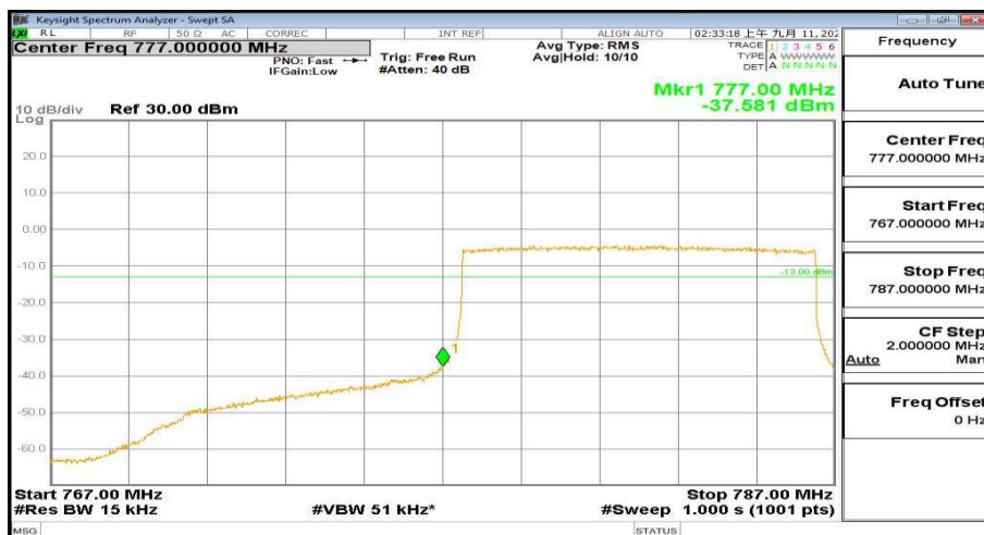
767MHz-787MHz_FreqLow_BW(10MHz)_RB(50@0)_QPSK_Band13
