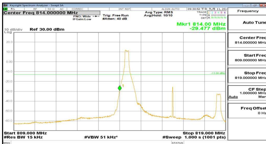
809MHz-819MHz_FreqLow_BW(_5MHz)_RB(1@0)_QPSK_Band26
