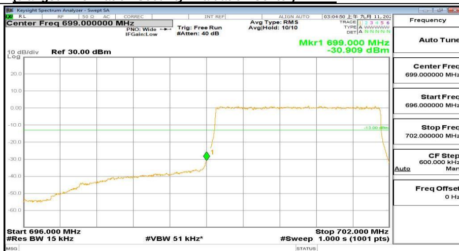
696MHz-702MHz_FreqLow_BW(3MHz)_RB(15@0)_QPSK_Band12
