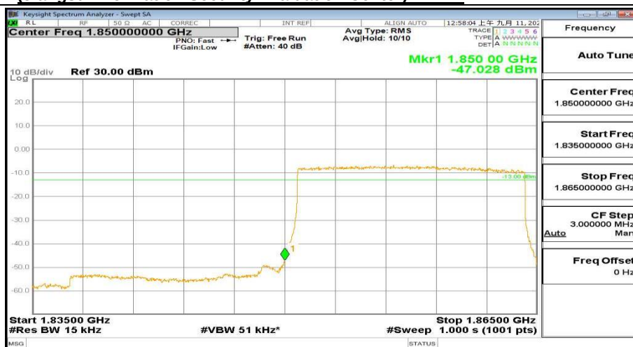
1835MHz-1865MHz_FreqLow_BW( 15MHz)_RB(75@0)_QPSK_Band25
