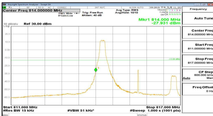
811MHz-817MHz_FreqLow_BW(3MHz)_RB(1@0)_QPSK_Band26
