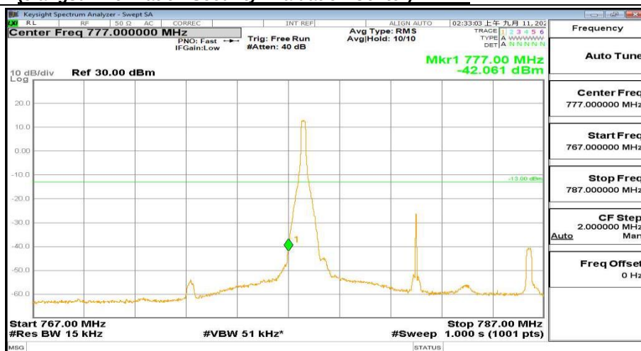
767MHz-787MHz_FreqLow_BW(10MHz)_RB(1@0)_QPSK_Band13
