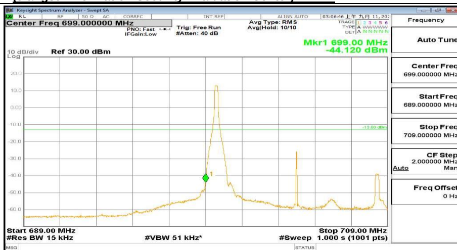
689MHz-709MHz_FreqLow_BW(10MHz)_RB(1@0)_QPSK_Band12
