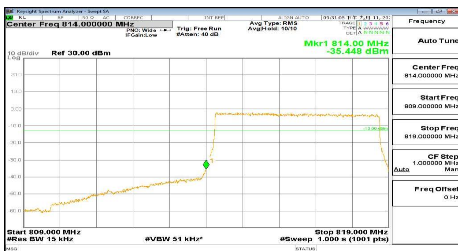
809MHz-819MHz_FreqLow_BW(_5MHz)_RB(25@0)_QPSK_Band26
