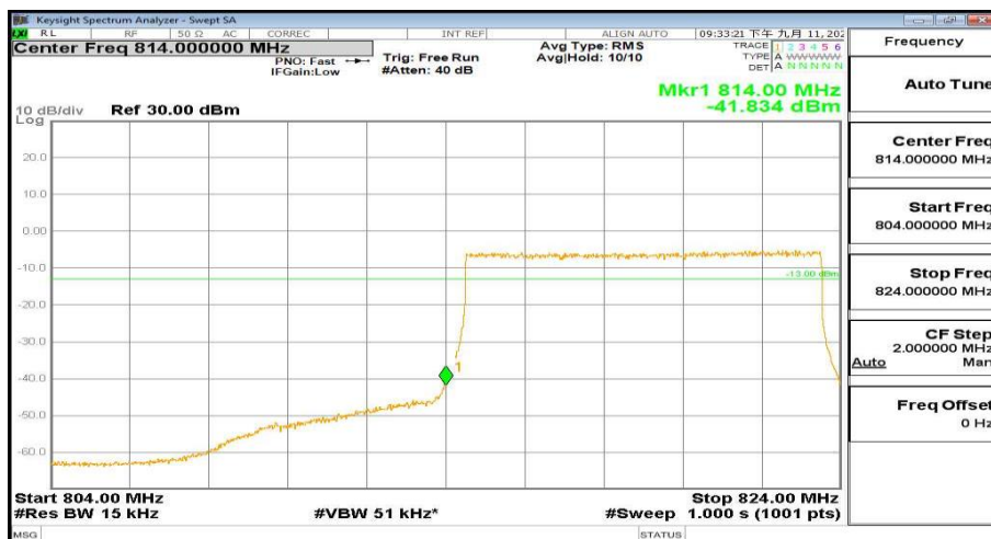
804MHz-824MHz_FreqLow_BW(10MHz)_RB(50@0)_QPSK_Band26
