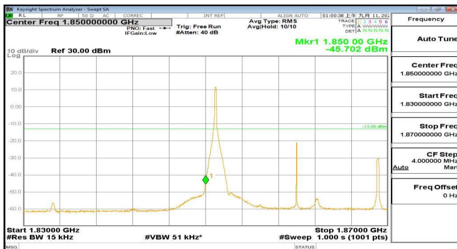
1830MHz-1870MHz_FreqLow_BW( 20MHz)_RB(1@0)_QPSK_Band25
