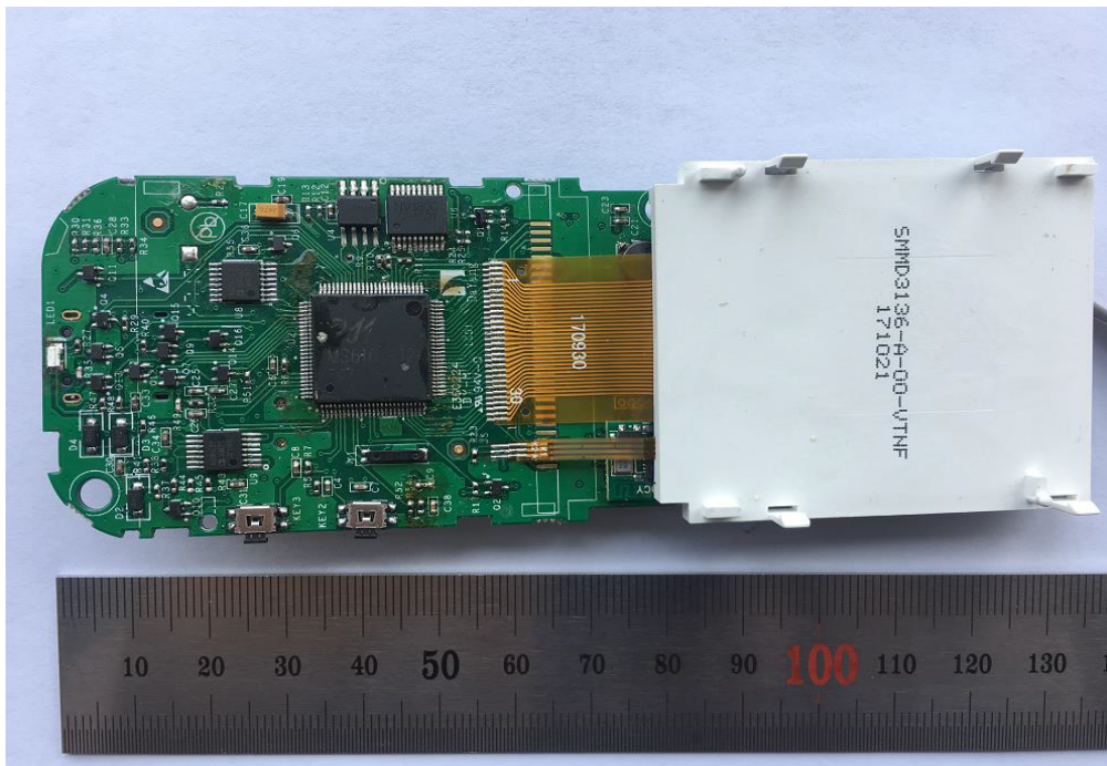
(4) EUT Photo
