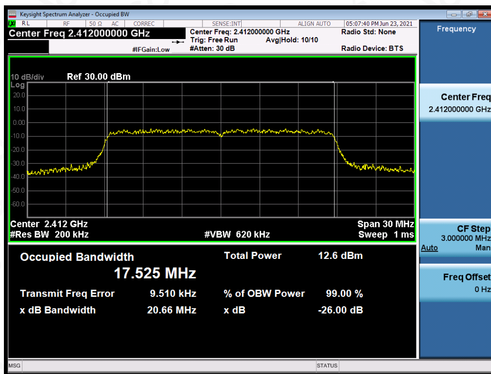
Test_Graph_802.11n20_ANT1_2412_MCS0_OBW
