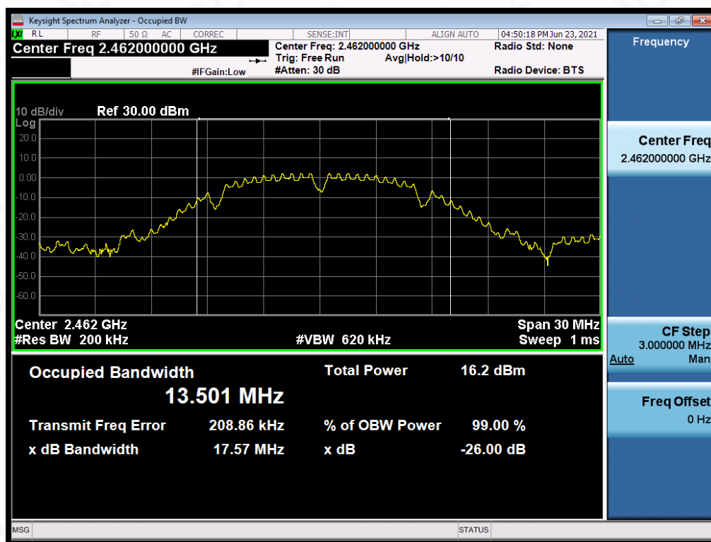
Test_Graph_802.11b_ANT1_2462_1Mbps_OBW
