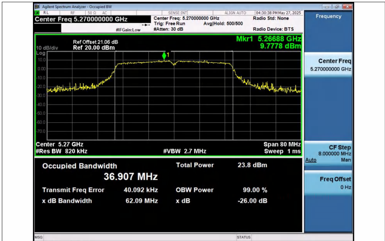
11N40SISO-Ant1-5270
