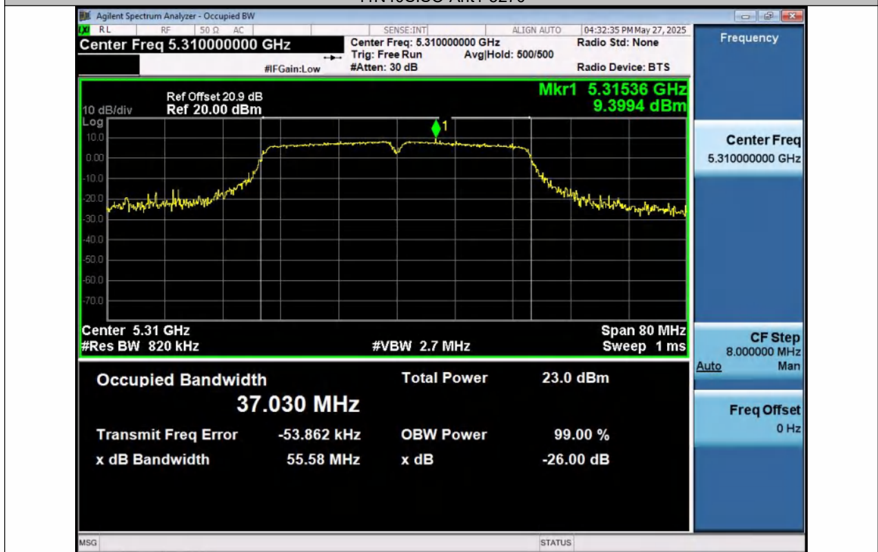
11N40SISO-Ant1-5310
